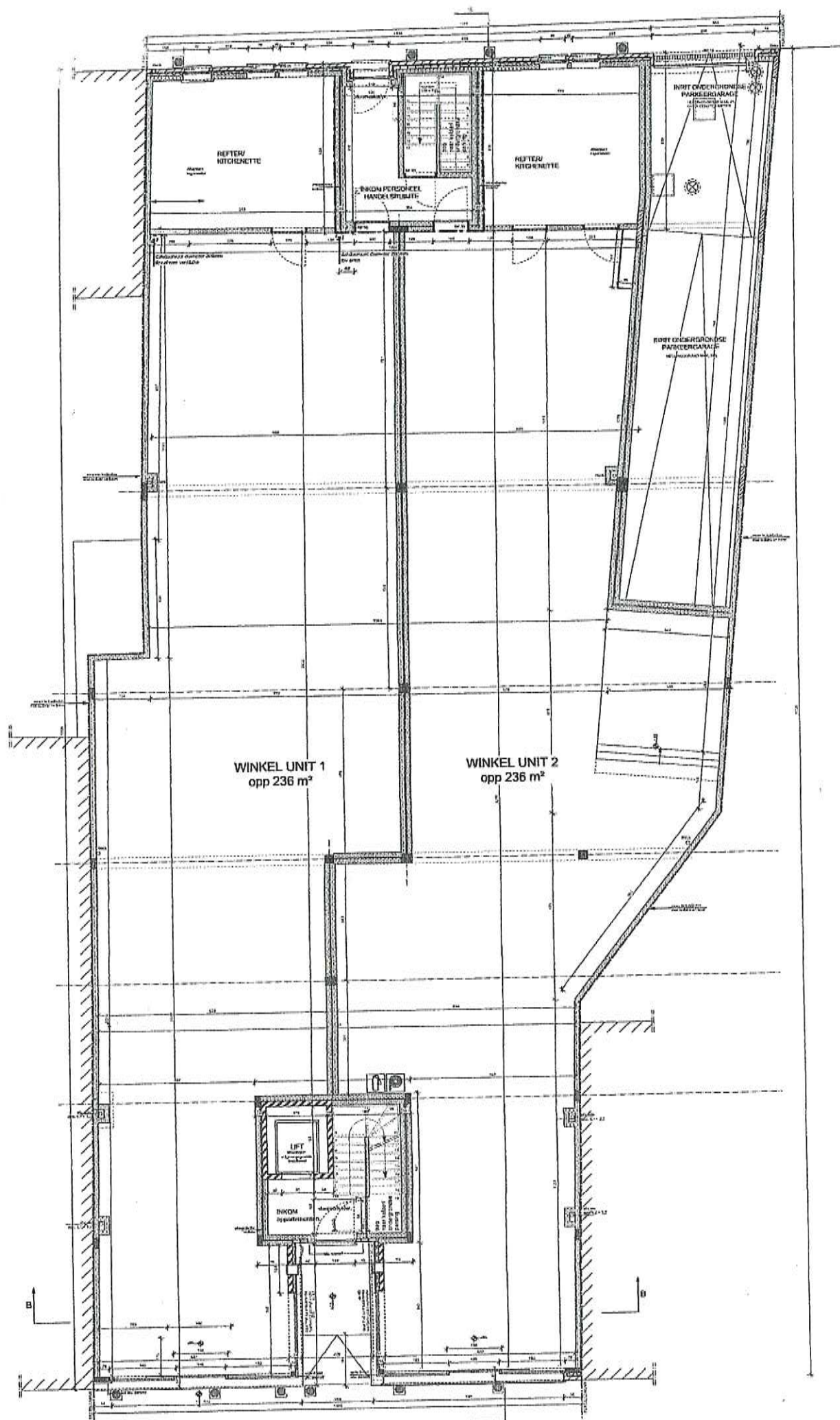
GELIJKVLOERS, schaal 1/50 Verkrijgbaar op: L.V. architecten Adviesbureau en Technisch Bureau
