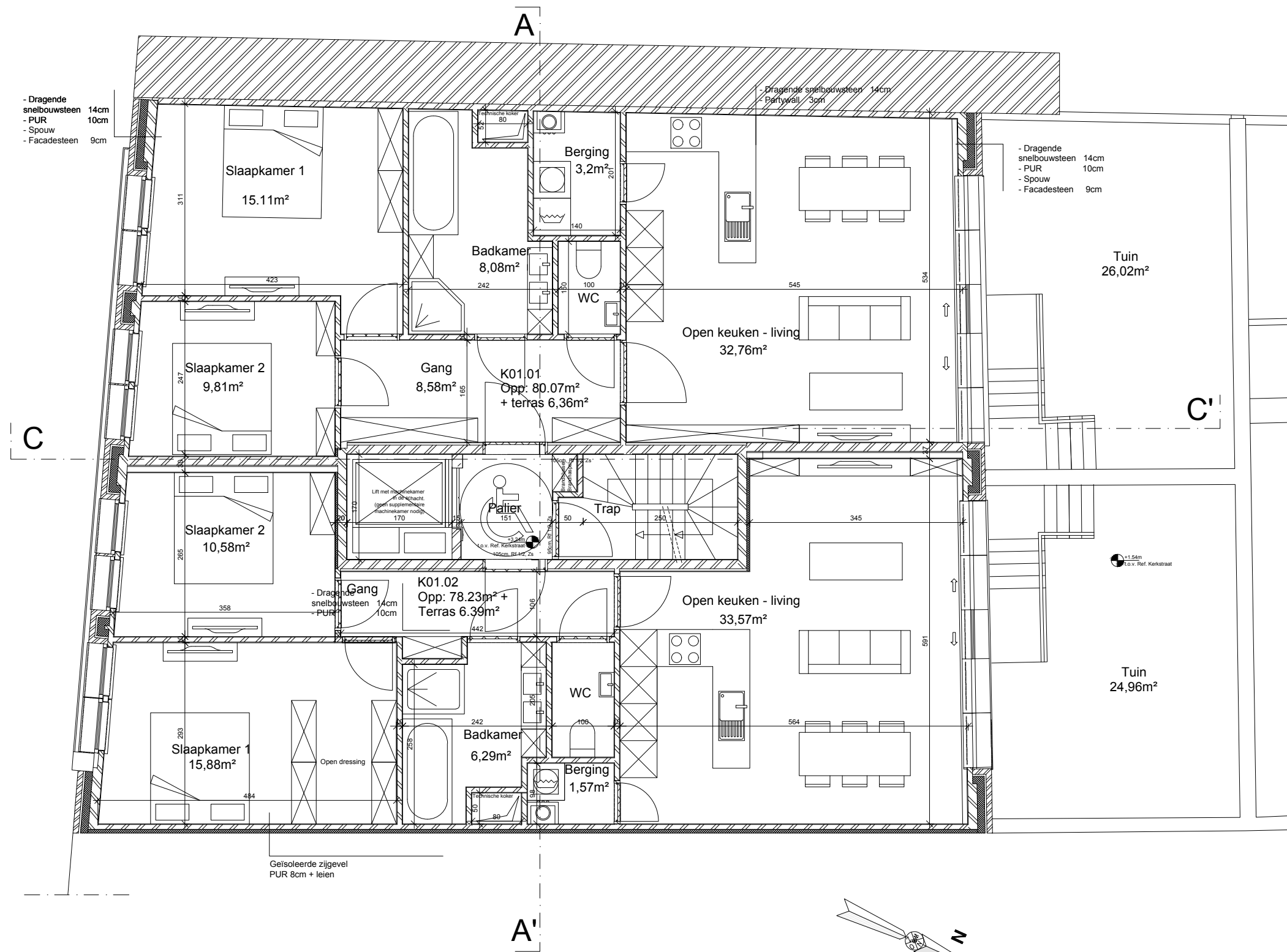
Plan verdieping +1 kerkstraat Schaal 1:75
