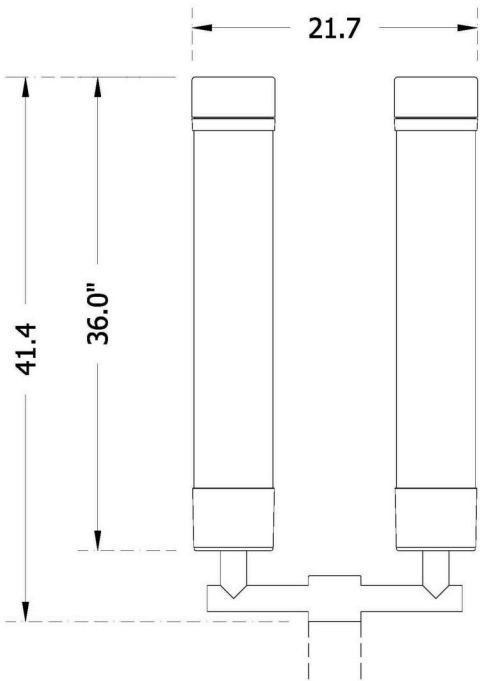
2 Arm Mount (2A)
