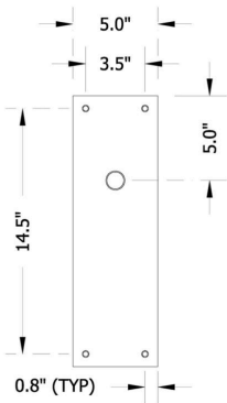
TA-SCR (Wall Bracket)
