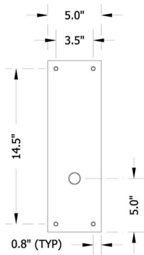
TA-SCU (Wall Bracket)
