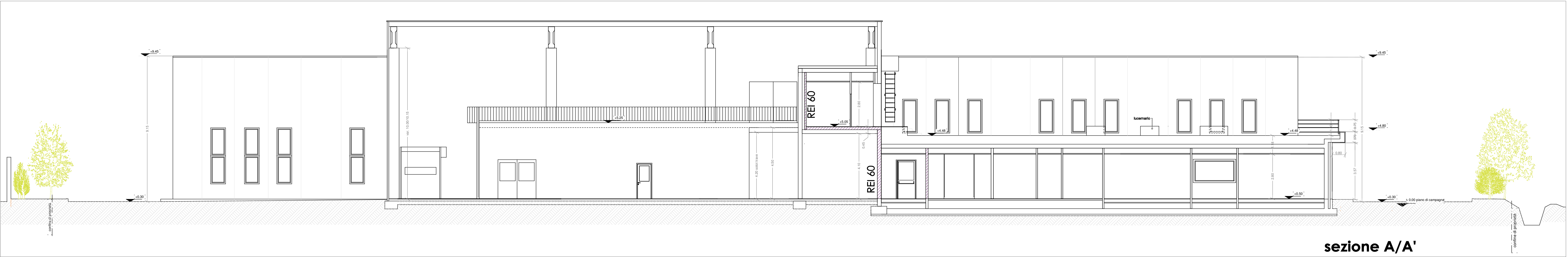
sezione A/A'
