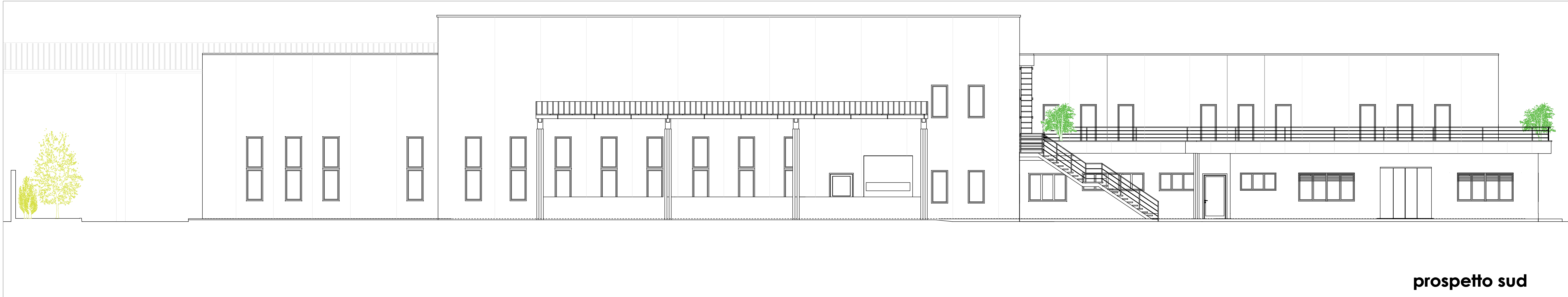
prospetto sud
