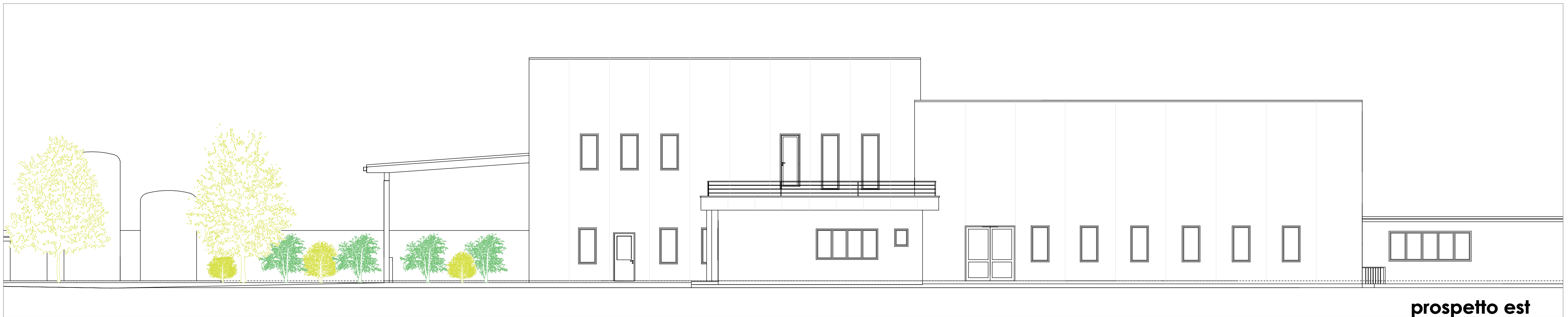
prospetto est
