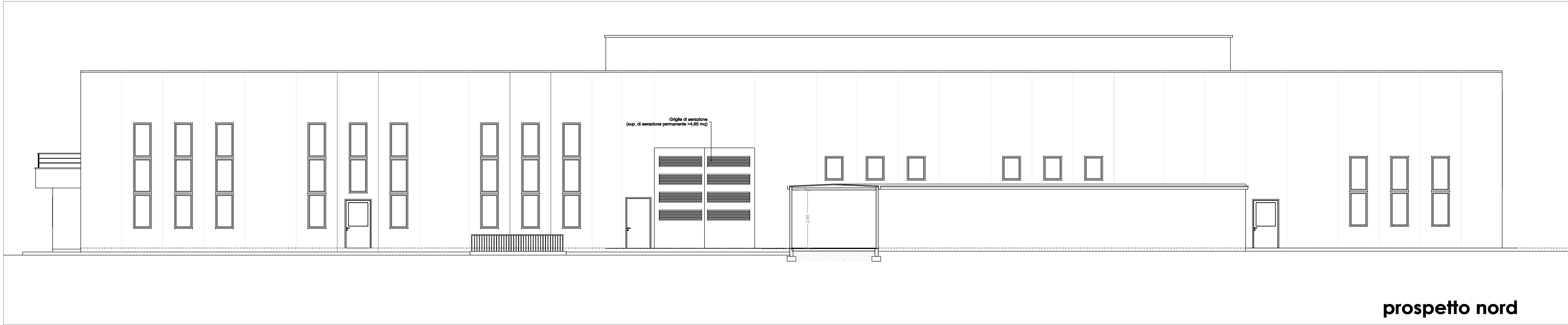
prospetto nord
