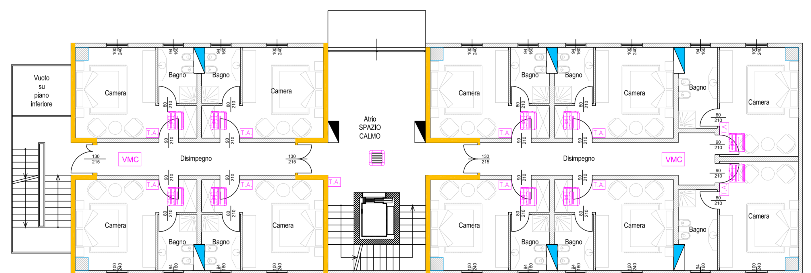
PIANTA PIANO SECONDO SCALA 1:100
