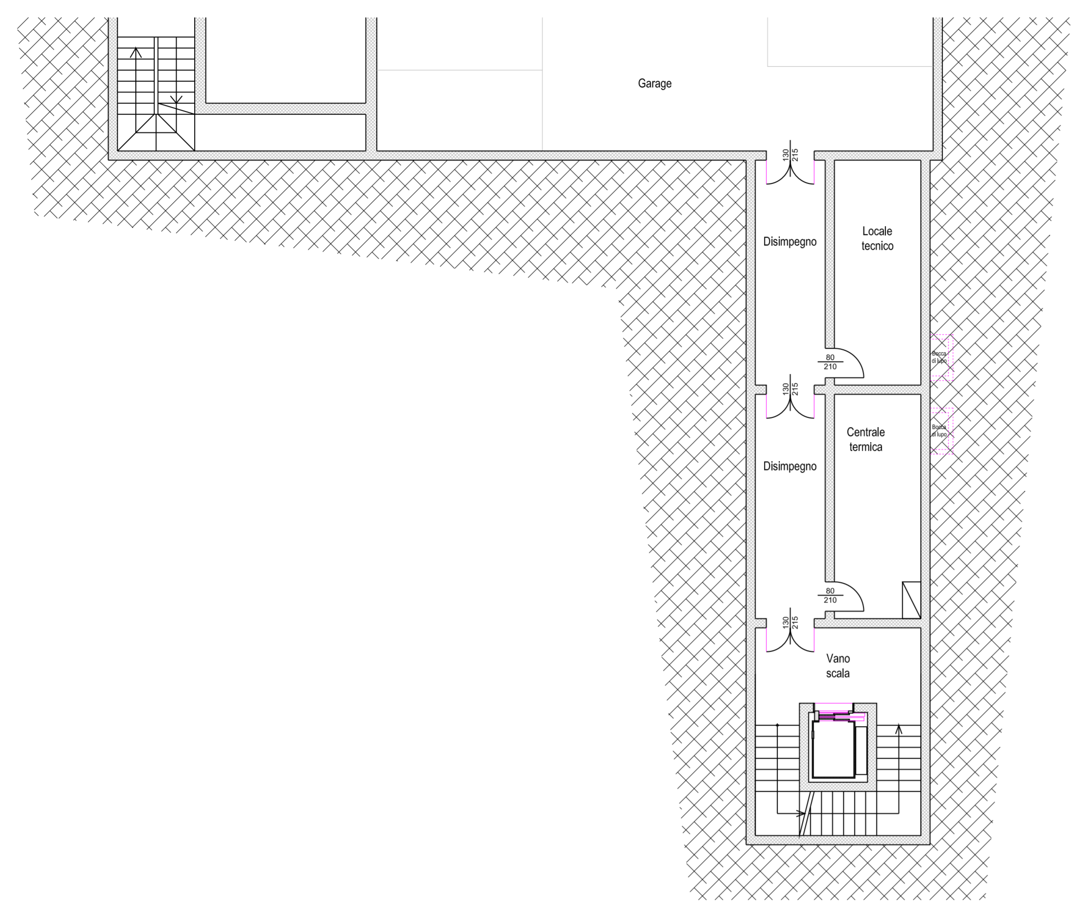
PIANTA SEMINTERRATO SCALA 1:100
