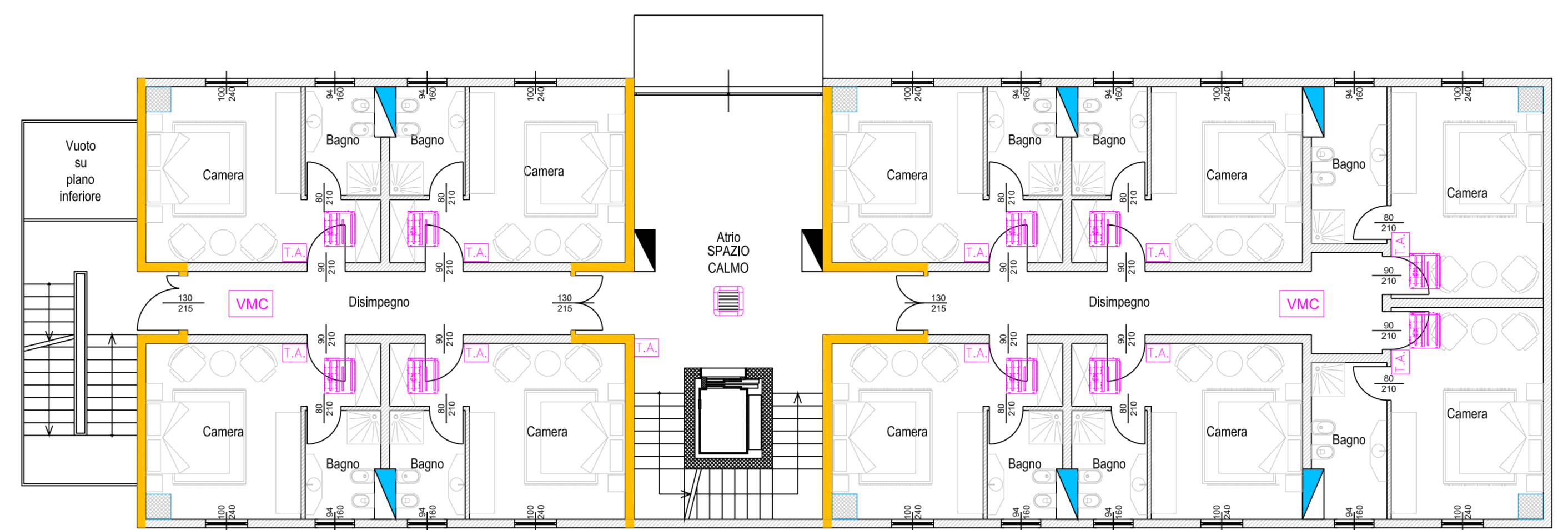
PIANTA PIANO PRIMO SCALA 1:100
