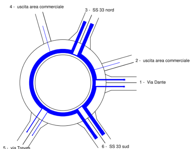
Figura 20 Rotatoria 2: Grafo flussi veicolari scenario di progetto
