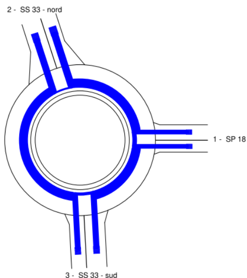
Figura 23 Intersezione 1: Grafo flussi veicolari scenario di progetto
