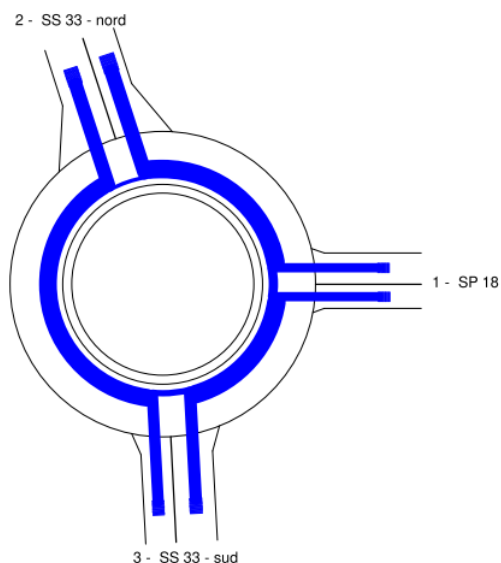
Figura 17 Rotatoria 1: Grafo flussi veicolari scenario di progetto
