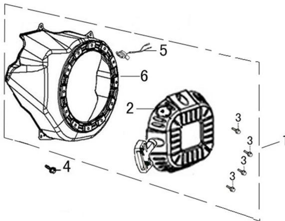
G210FA-C スターター(STARTER SUBASSEMBLY)
