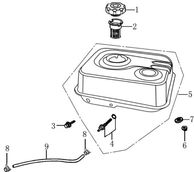
G210FA-C 燃料タンク(FUEL TANK)
