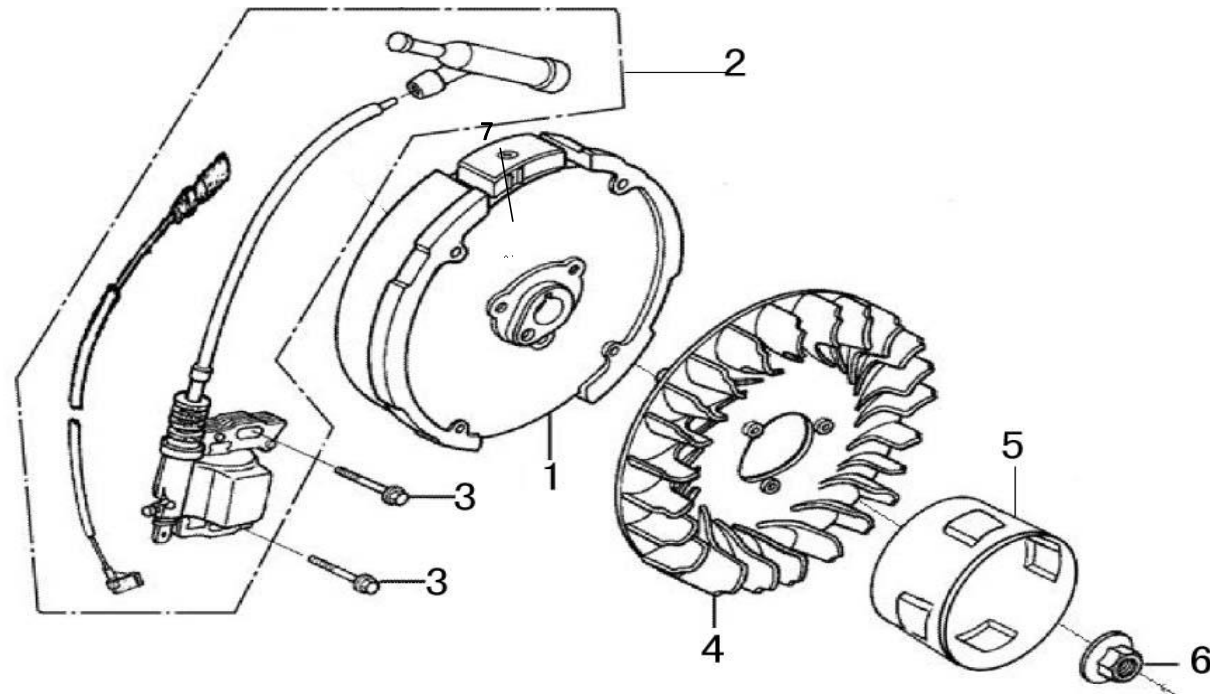
G210FA-C フライホイール/点火コイル(FLYWHEEL/COIL ASSY.)
