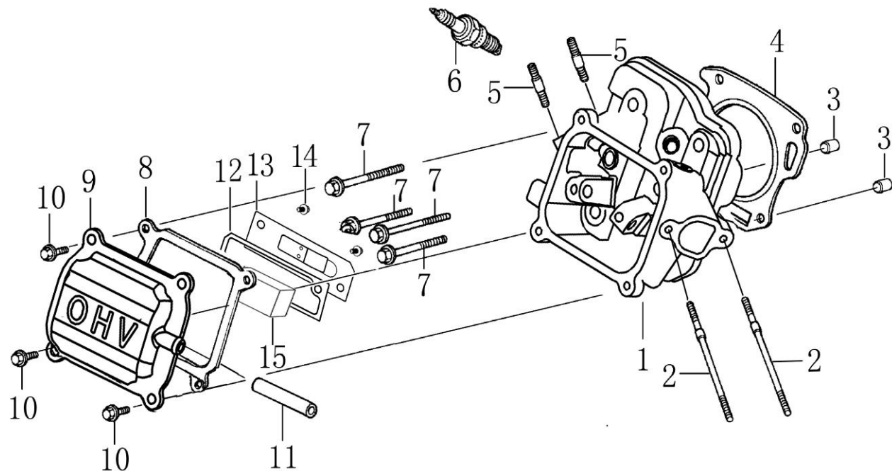
G210FA-C シリンダヘッド(CYLINDER HEAD)
