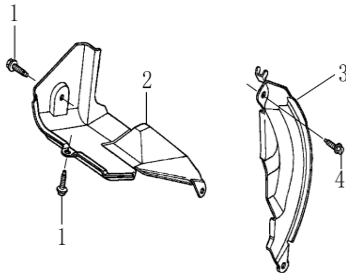
G210FA-C 導風部(DIVERSION ASSY.)
