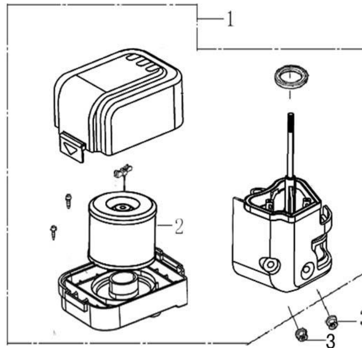
G210FA-C エアークリーナー(AIR CLEANER)
