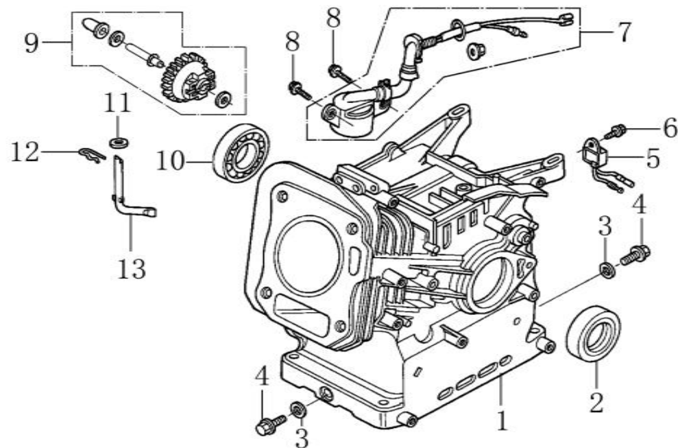
G210FA-C クランクケース(CRANK CASE)
