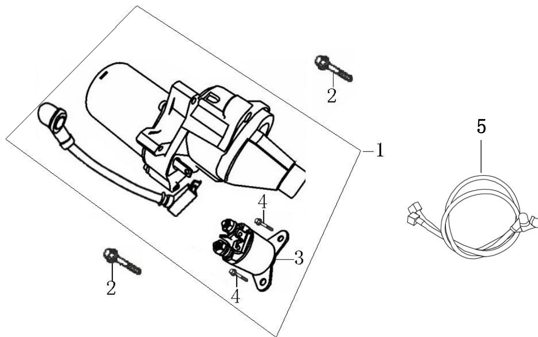
MSB28N スターティングモーター (STARTER MOTOR)
