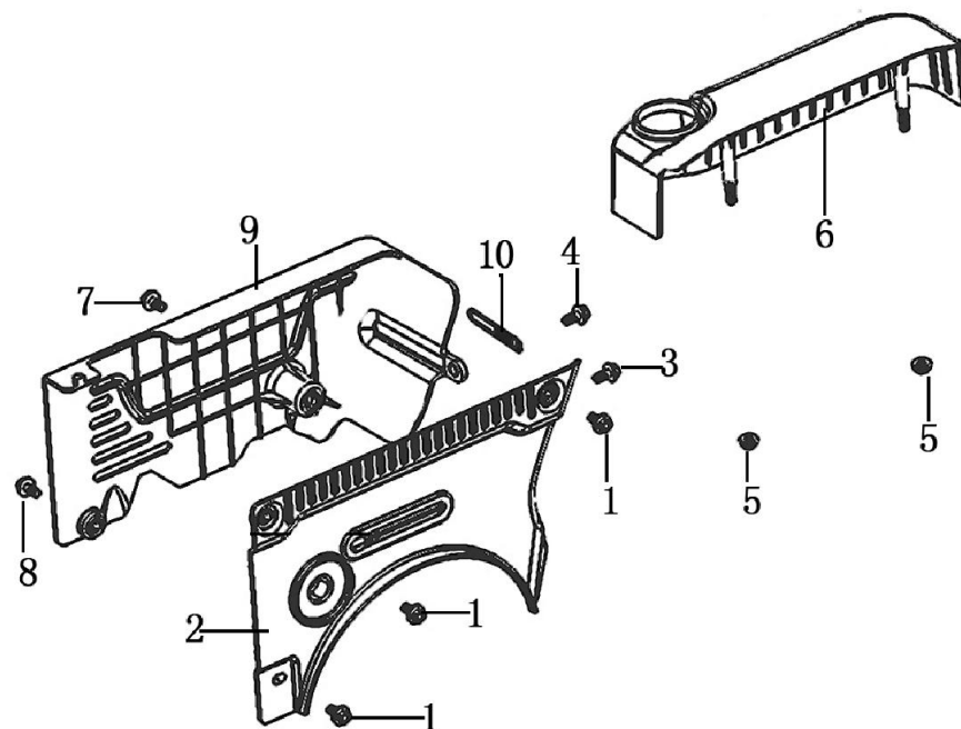
MSB28N カバー (Cover)
