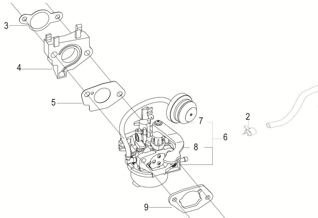
MSB28N キャブレター (CARBURETOR)
