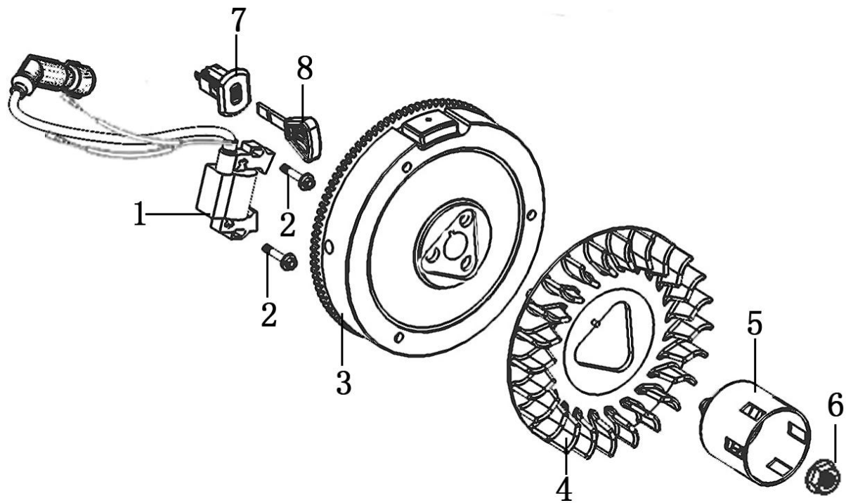
MSB28N フライホイール (FLYWHEEL/COIL ASSY.)
