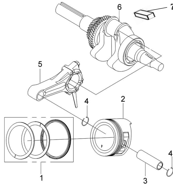
MSB28N クランクシャフト/ピストン (CRANKSHAFT/PISTON)
