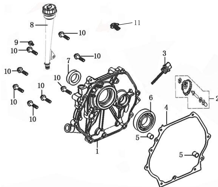
MSB28N クランクケースカバー (CRANK CASE COVER)
