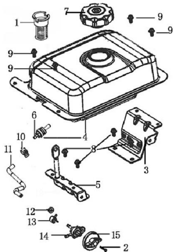
MBS28N 燃料タンク(FUEL TANK)
