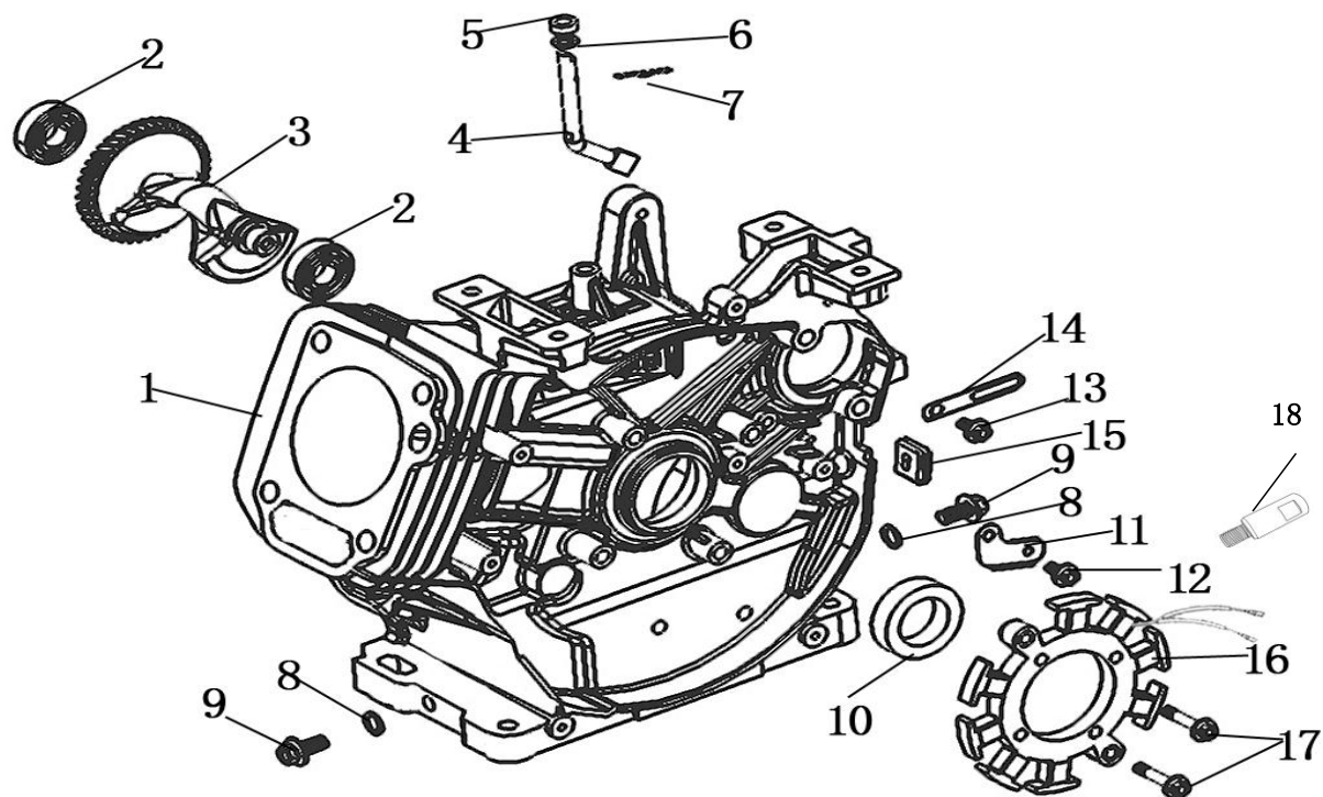
MSB28N クランクケース(CRANK CASE)
