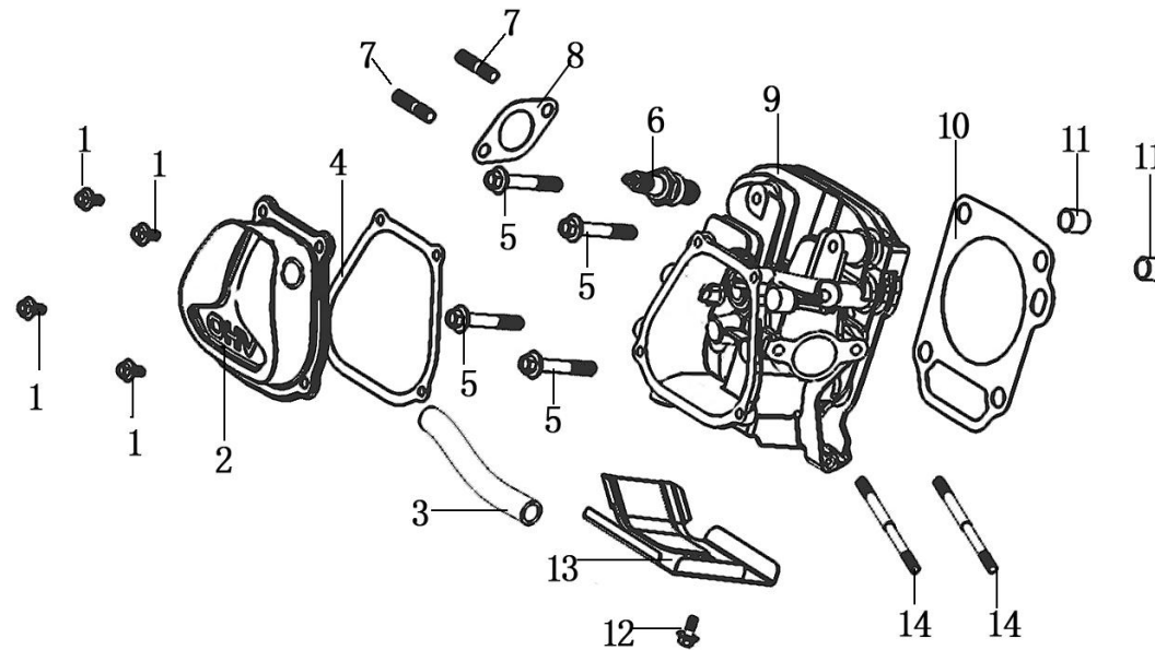
MSB28N シリンダヘッド(CYLINDER HEAD)
