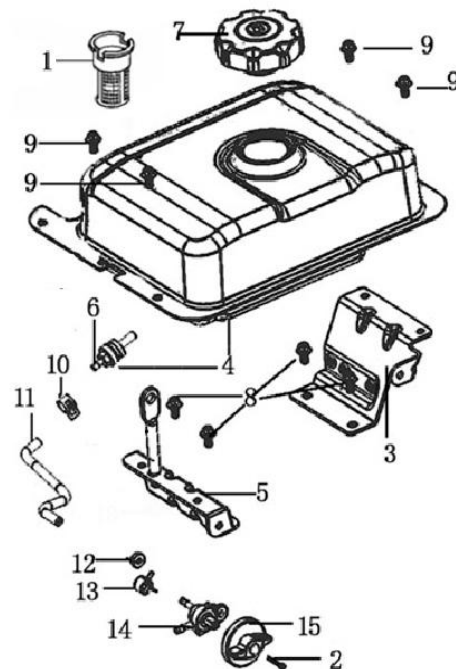
MSB28N 燃料タンク(FUEL TANK)
