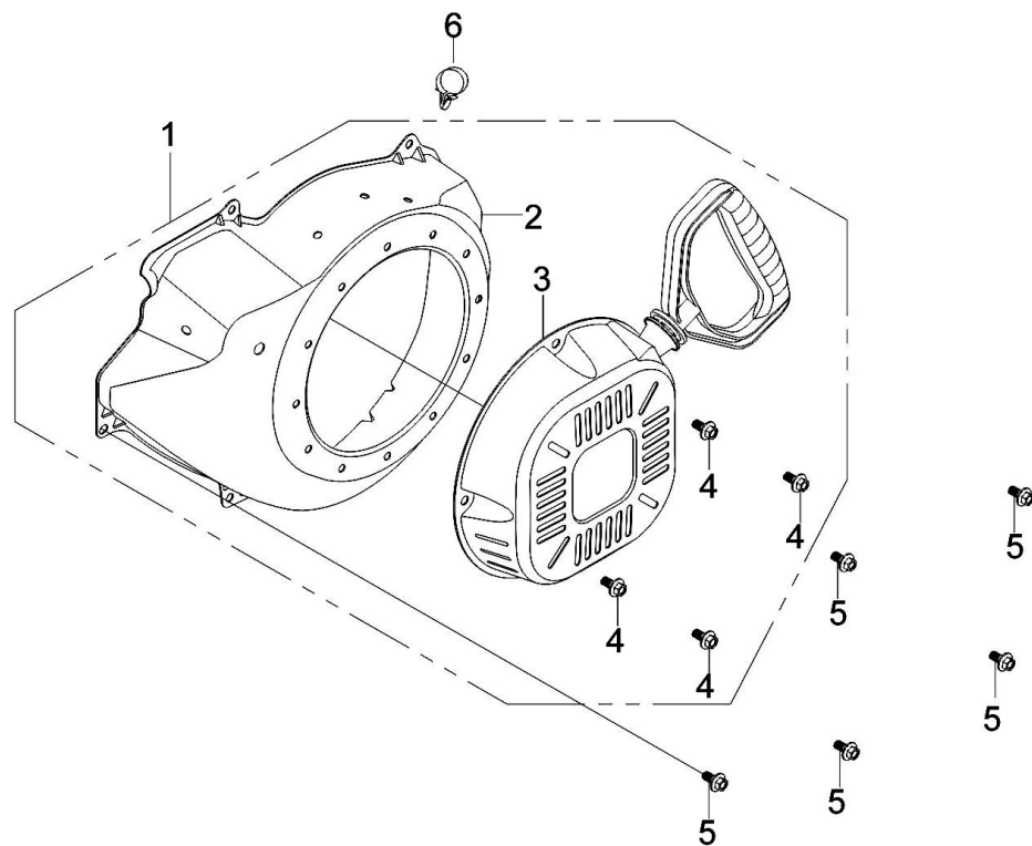
MSB28N リコイルスターター (STARTER SUBASSEMBLY)
