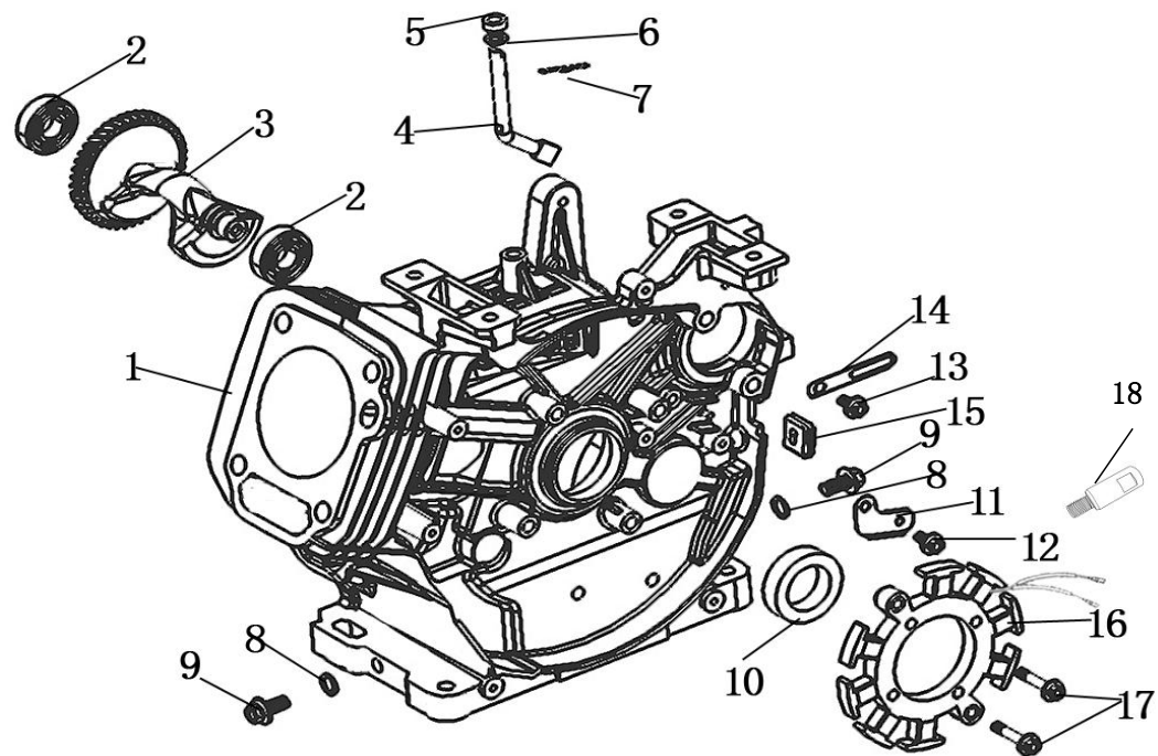
MSB28N クランクケース(CRANK CASE)
