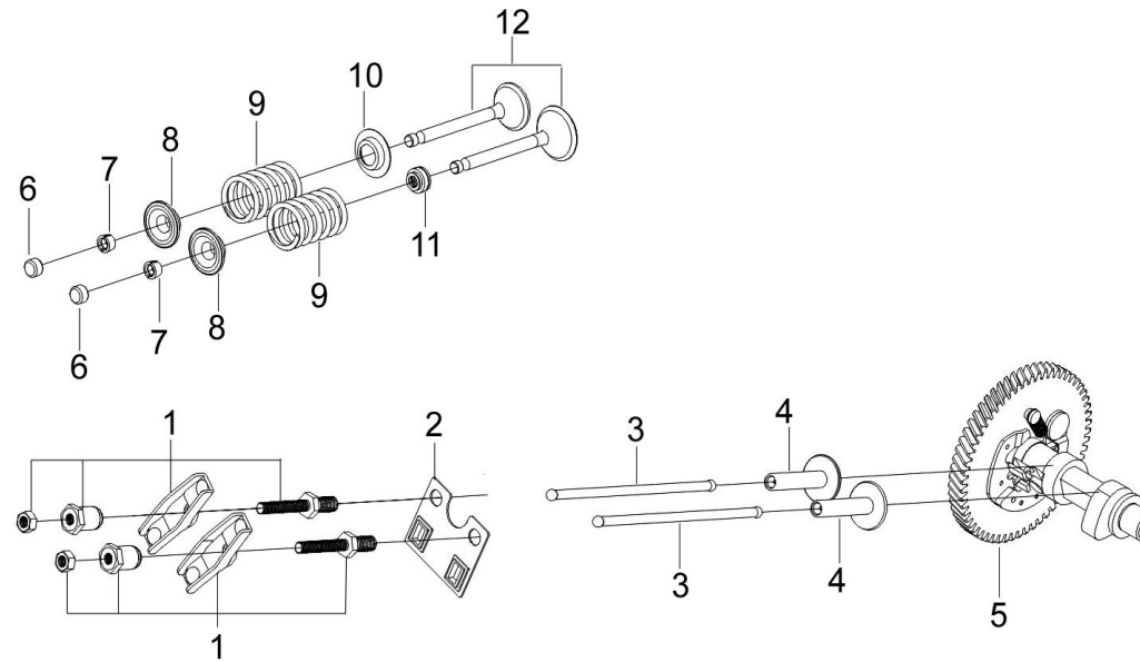
MSB28N カムシャフト(GAS DISTRIBUTION ADJUSTMENT)
