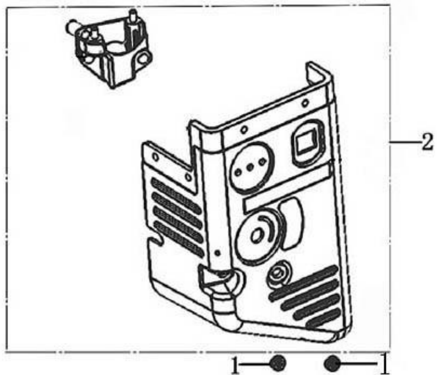
MSB28N エアークリーナー (AIR CLEANER)
