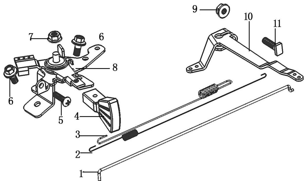
MSB28N コントロール (CONTROL SYSTEM)
