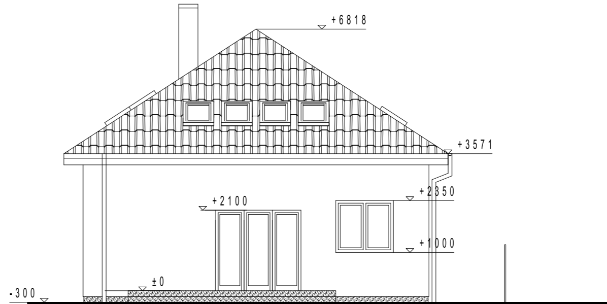
POHLED jižní - ze zahrady 1:100
