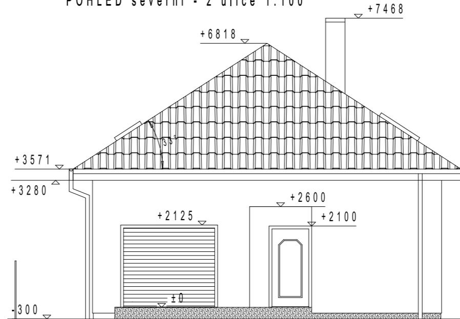
POHLED severní - z ulice 1:100
