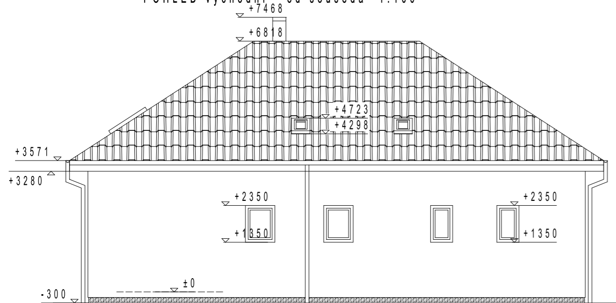
POHLED východní - od souseda 1:100
