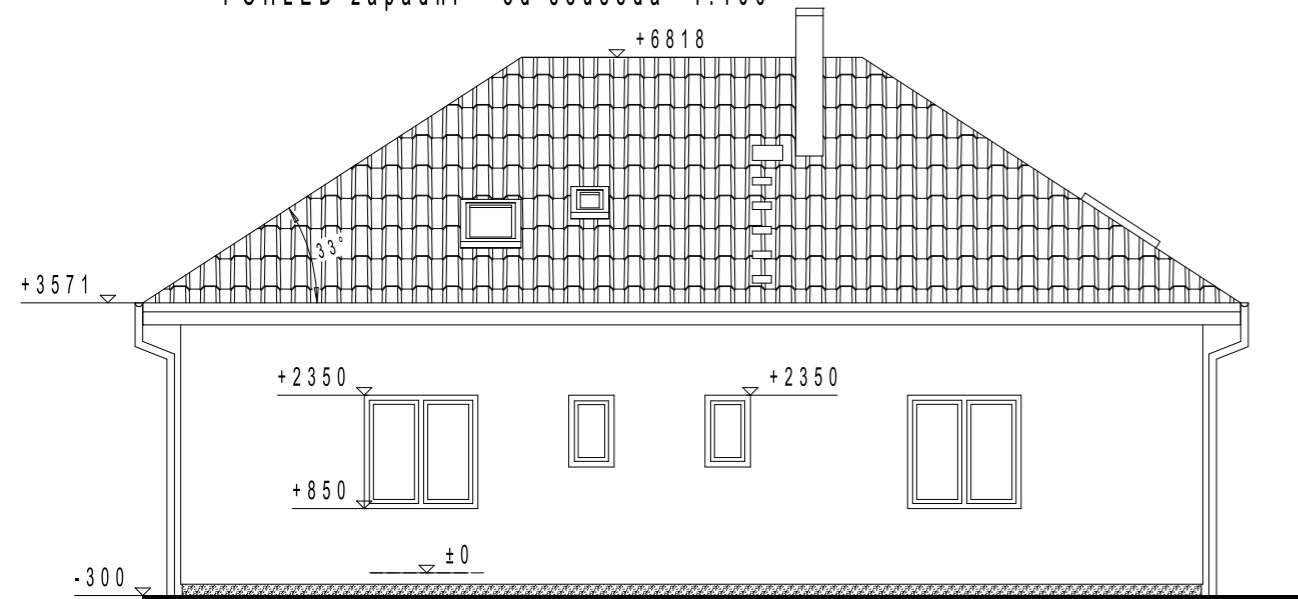
POHLED západní - od souseda 1:100
