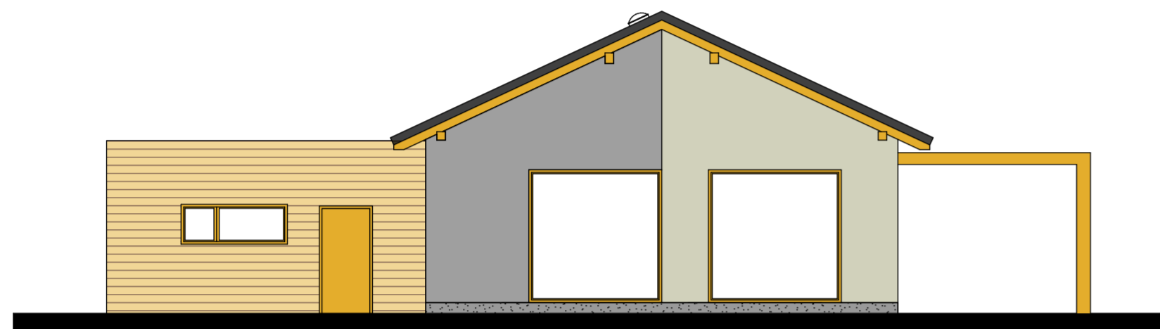
JIHOVÝCHODNÍ POHLED
