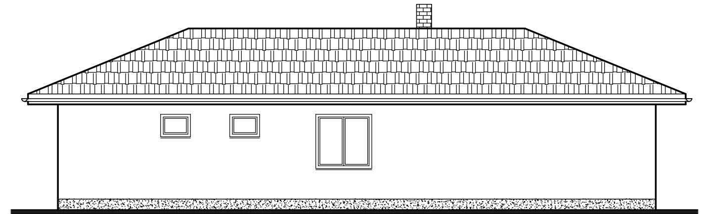
POHLED SEVERNÍ
