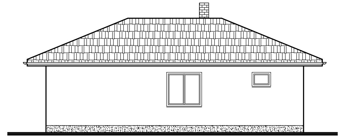
POHLED VÝCHODNÍ
