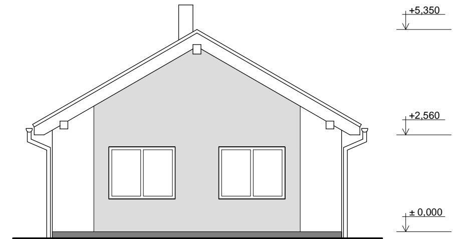
POHLED ČELNÍ = POHLED ZADNÍ
