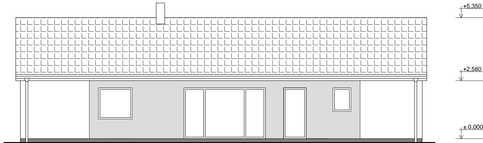
POHLED BOČNÍ II
