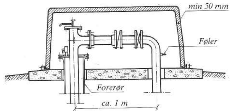
snit B-B
