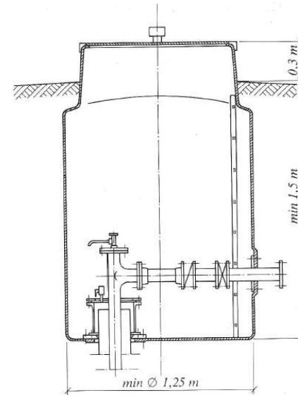
snit A-A
