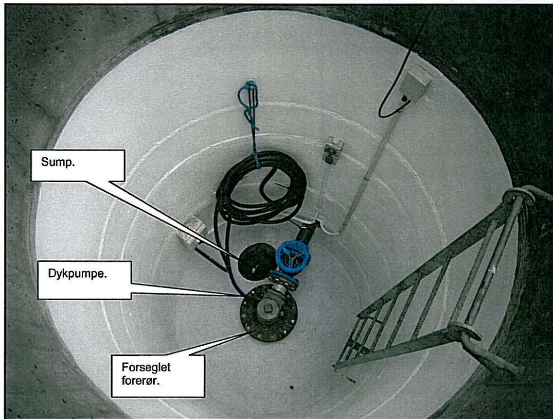
Fig. 21: Tørbrønd med boring med forseglet forerør, dykpumpe og sump.
