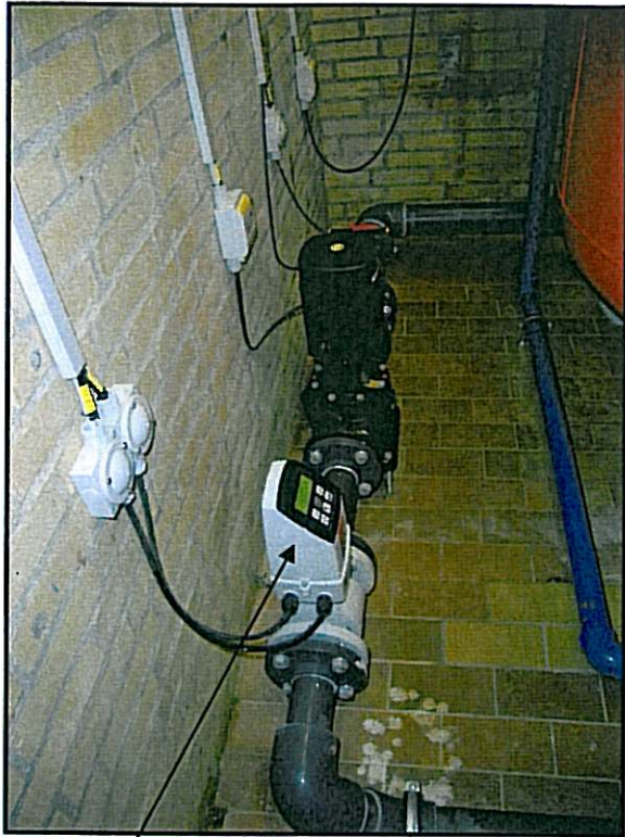
Fig. 18: Digital aflæsning af vandforbruget.
