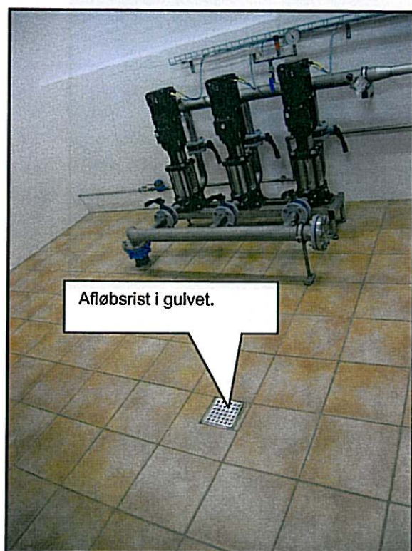
Fig. 10: Afløbsrist i gulvet er tilkoblet regnvandsledning.
