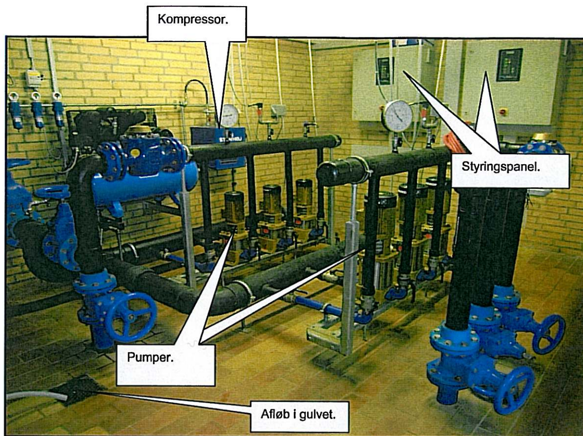
Fig. 15: Vandværket består af rentvandspumper, kompressor, styringspanel og afløb i gulvet. Rentvandspumpekapaciteten er på hver 9,5 \text{ m}^3/\text{h} . Afløbet i gulvet er tilkøbtet regnvandslednind.
