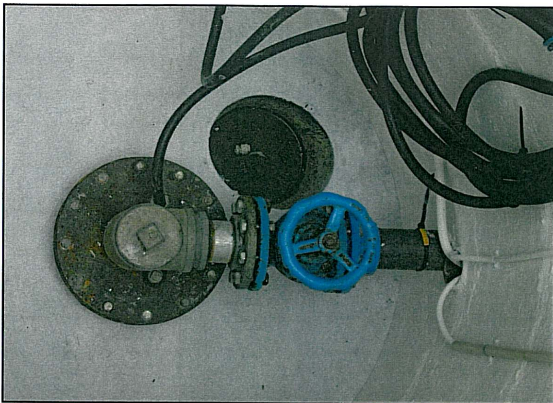
Fig. 22: Forseglet forerør.
