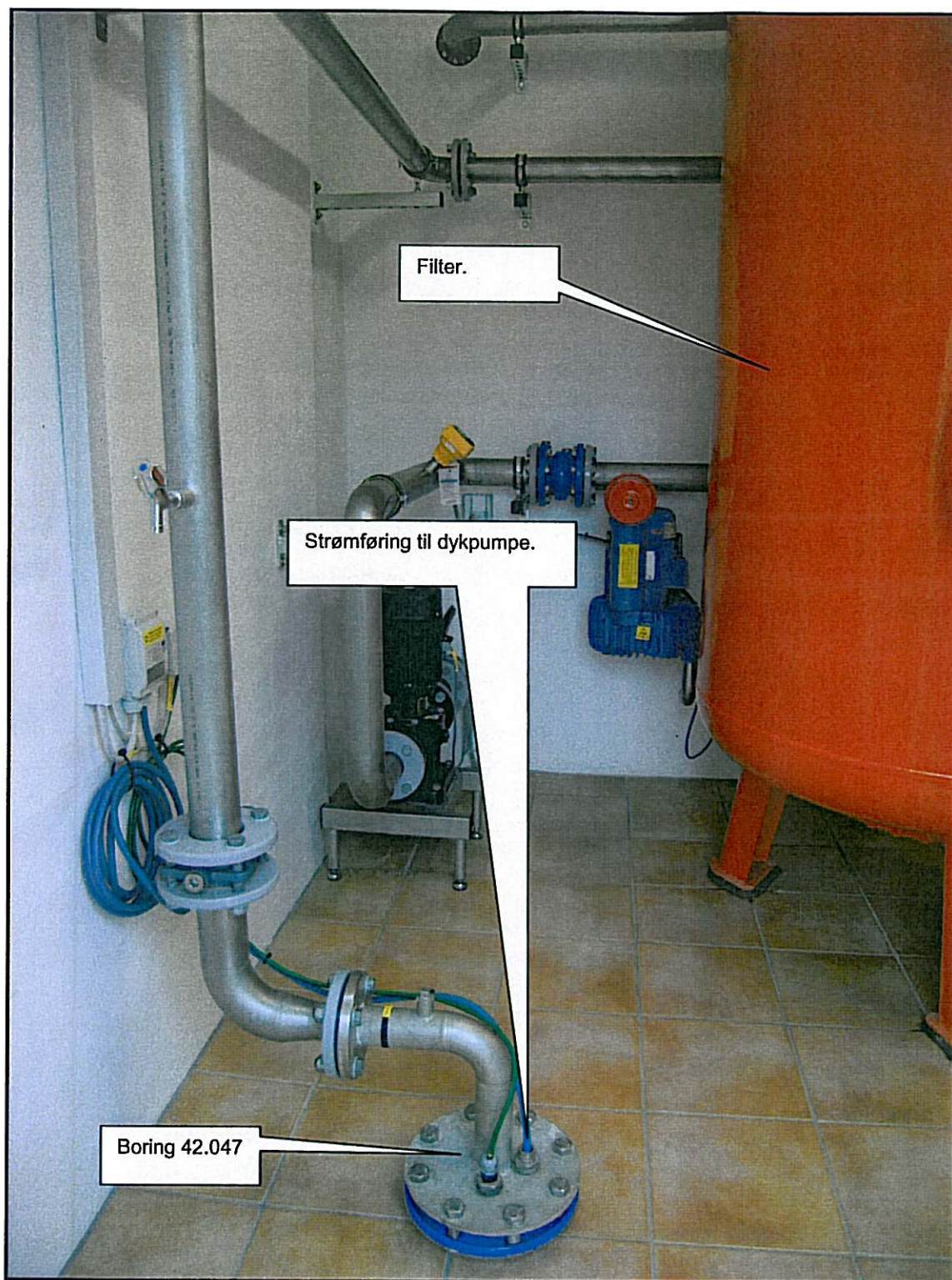
Fig. 7: Boring med dykpumpe og filter.
