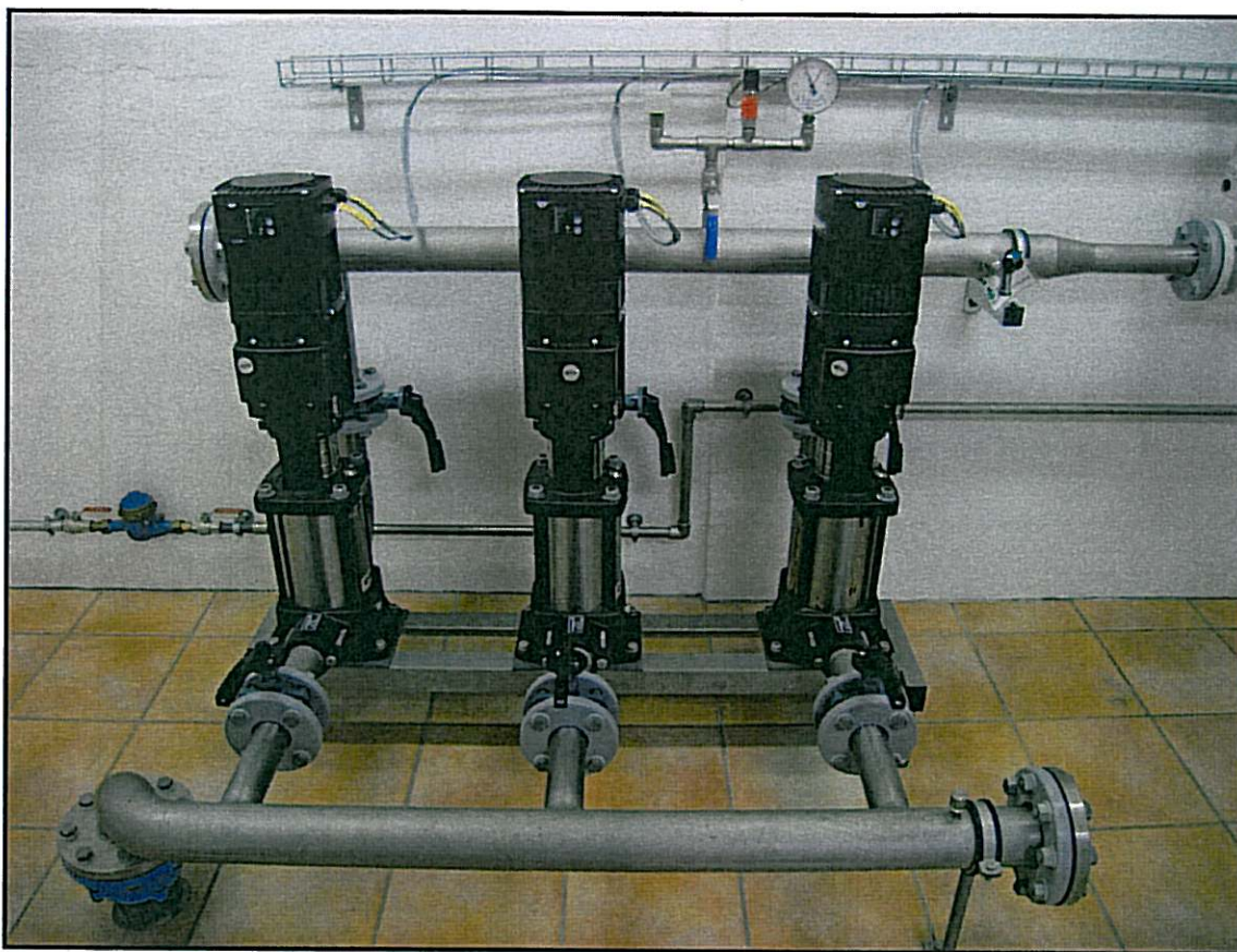
Fig. 9: Tre rentvandspumper med hver en kapacitet på 9,5 \text{ m}^3/\text{h} .
