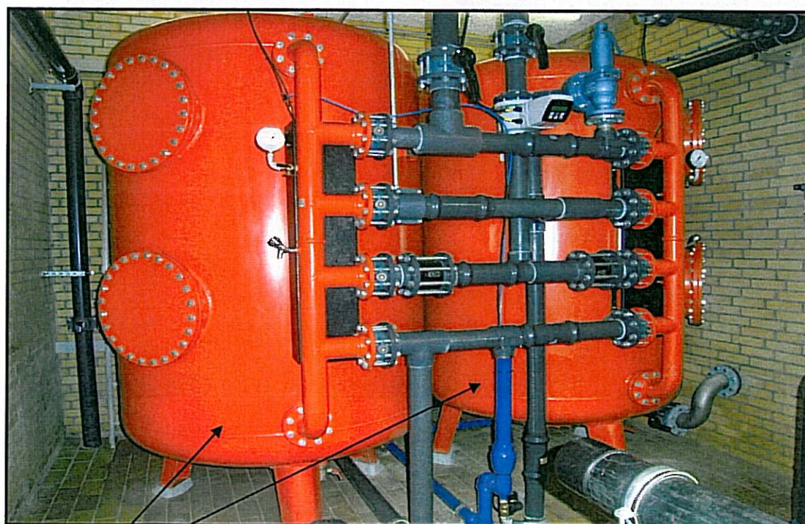
Fig. 16: Sandfiltre.
