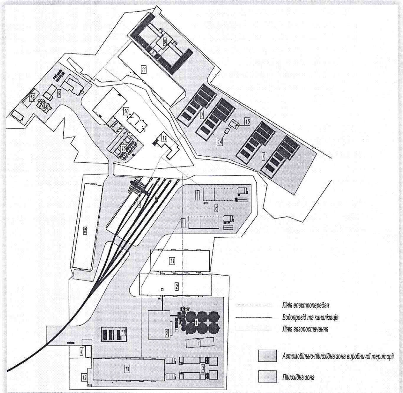
Мал. 7. Схема інженерних мереж індустріального парку.
