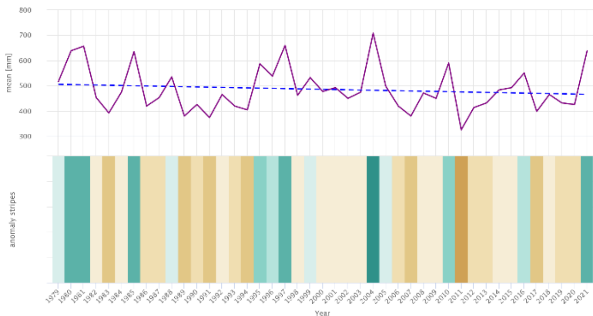
Рисунок 3.3 – Середньорічна кількість атмосферних опадів, тенденція і аномалії, 1979 – 2023 роки 11
