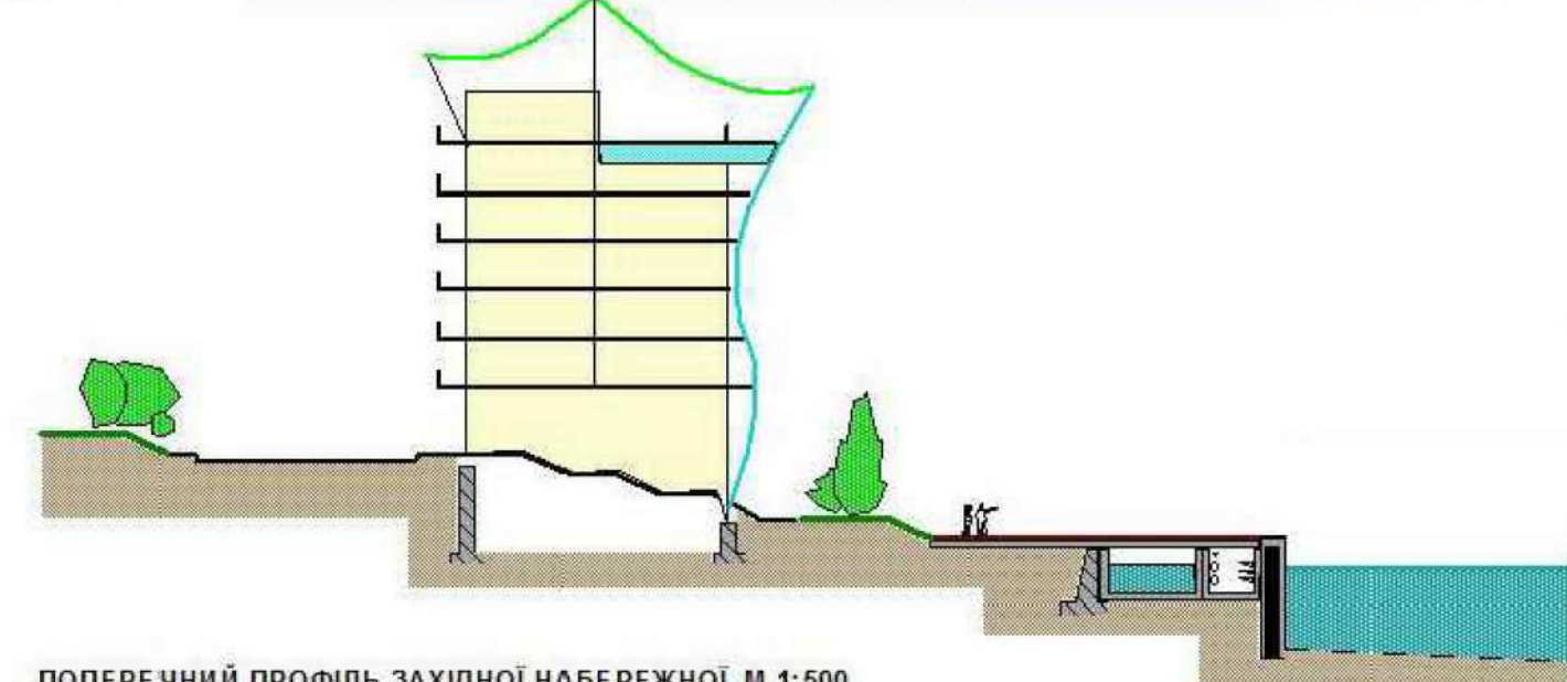
ПОПЕРЕЧНИЙ ПРОФІЛЬ ЗАХІДНОЇ НАБЕРЕЖНОЇ, М 1:500
