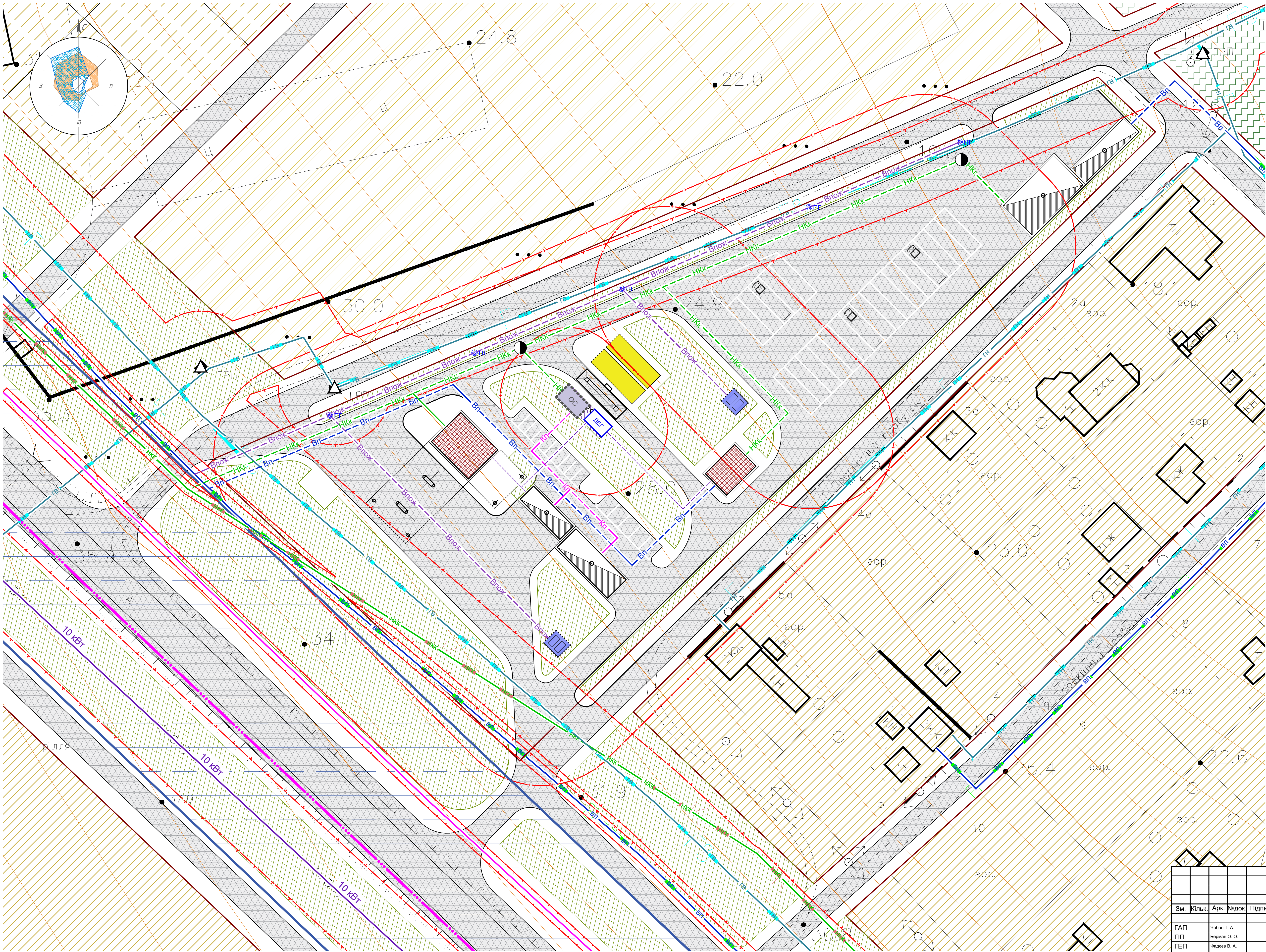
СХЕМА ІНЖЕНЕРНОГО ЗАБЕЗПЕЧЕННЯ ТЕРИТОРІЇ (М 1 : 500)
