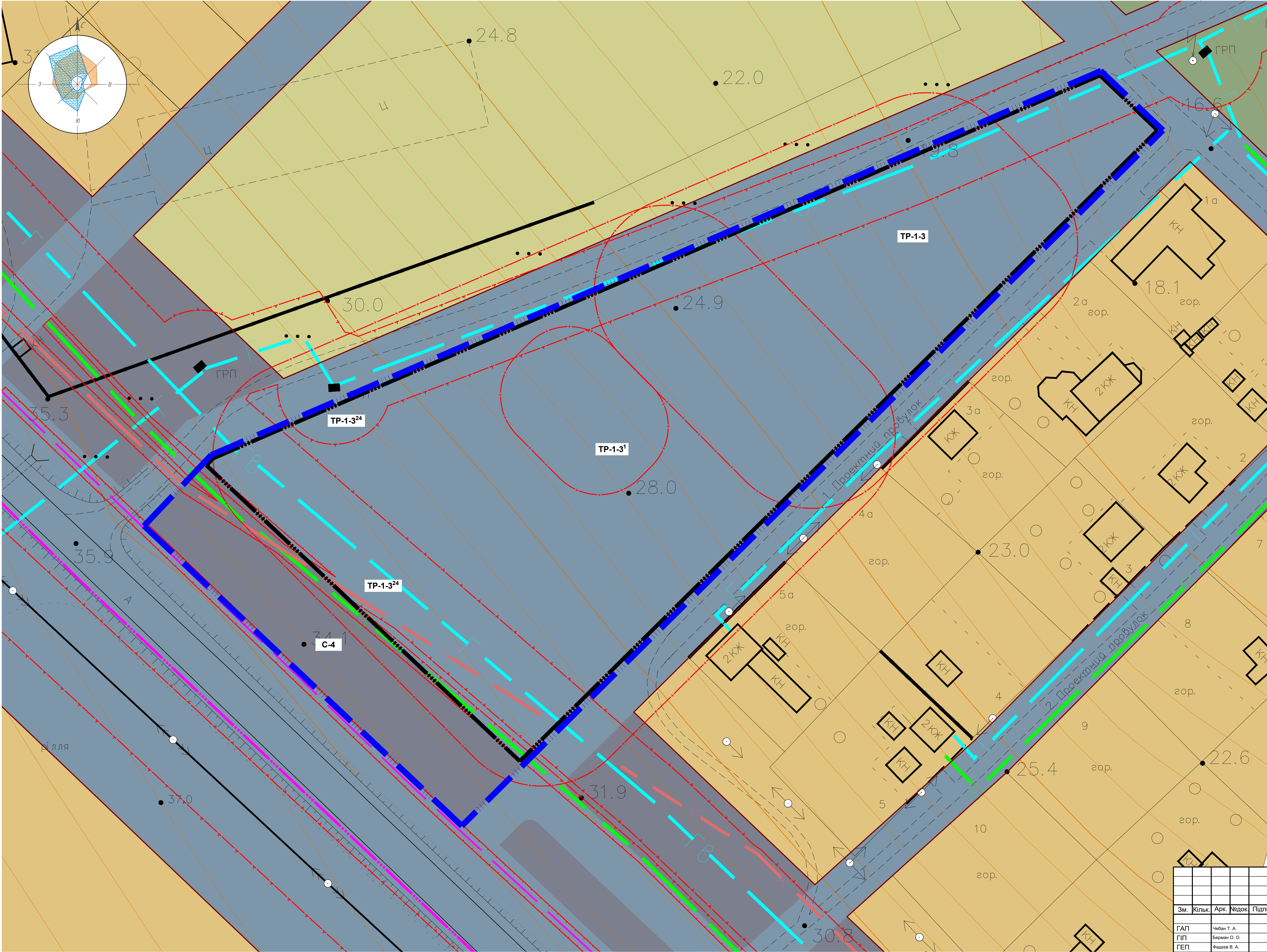
ПЛАН ФУНКЦІОНАЛЬНОГО ЗОНУВАННЯ ТЕРИТОРІЇ (М 1 : 500)
