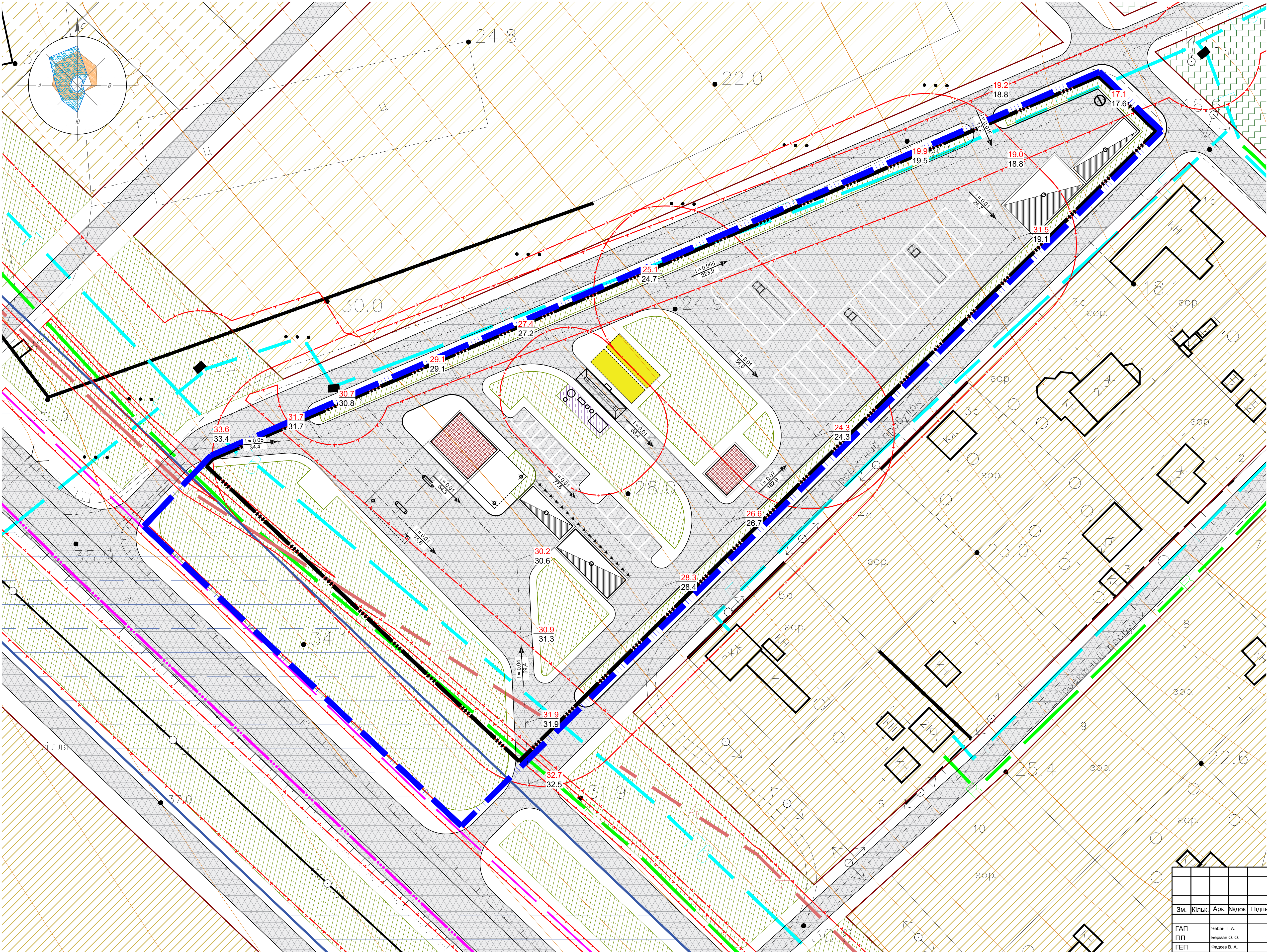
СХЕМА ІНЖЕНЕРНОЇ ПІДГОТОВКИ, БЛАГОУСТРОЮ ТЕРИТОРІЇ ТА ВЕРТИКАЛЬНОГО ПЛАНУВАННЯ (М 1 : 500)
