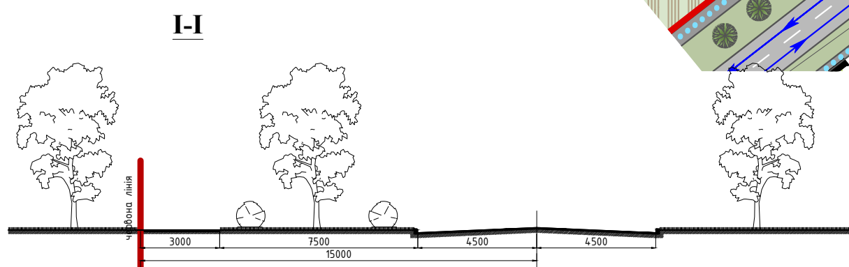
Поперечний профіль вулиці з червоними лініями М 1:200 I-I
