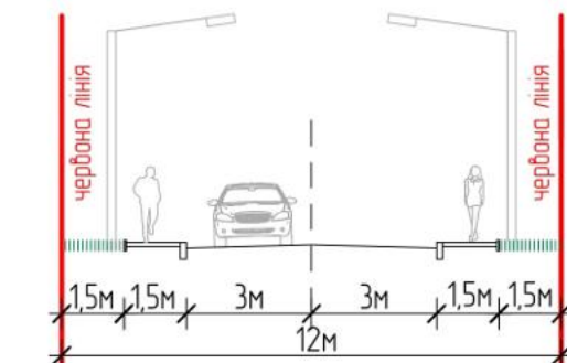
Поперечний профіль вул. Михайла Грушевського М 1:200
