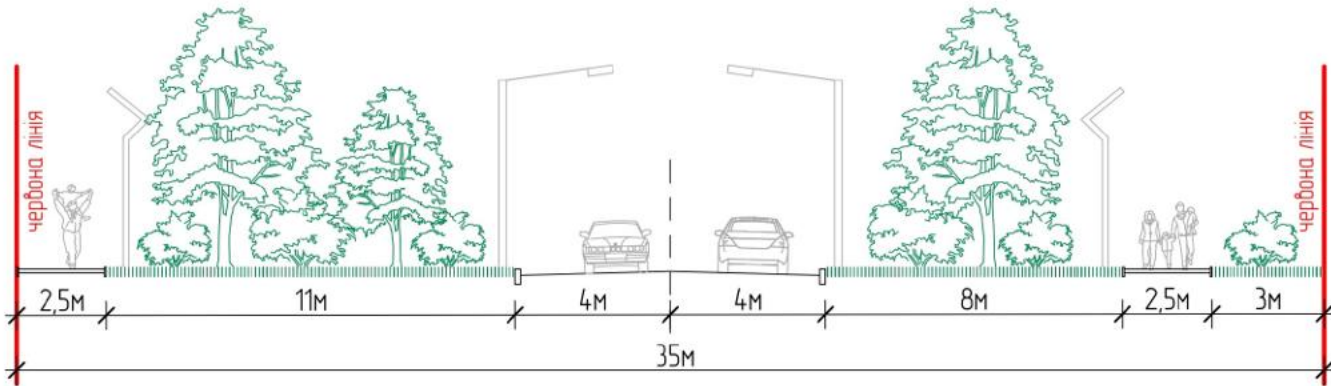
Поперечний профіль вул. Дмитра Яворницького М 1:200
