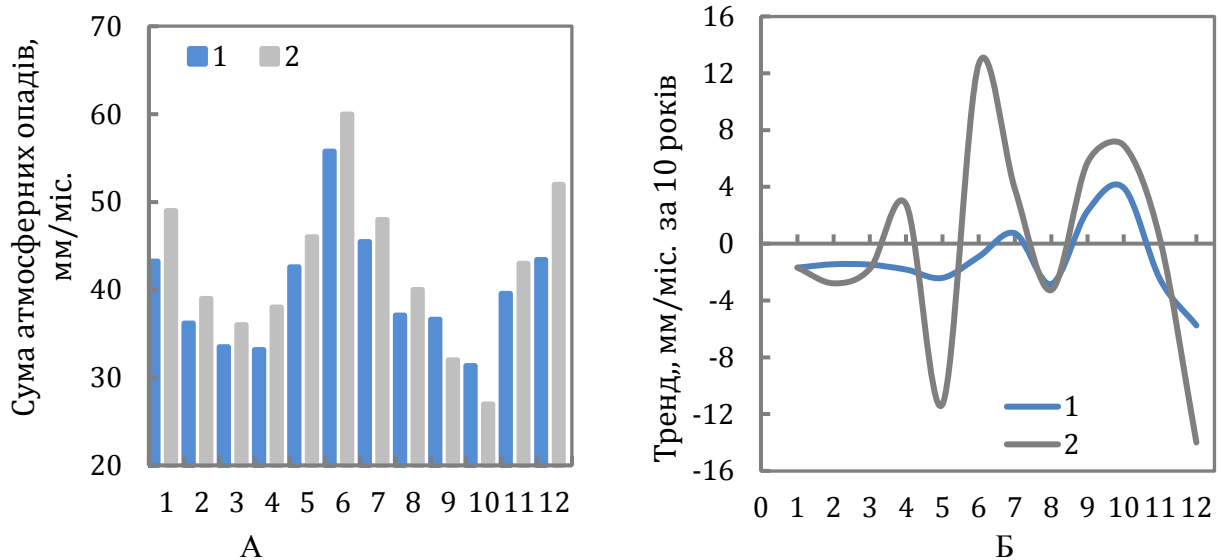
Рис. 4. Сезонний хід метеорологічної суми атмосферних опадів (А) та тенденції його змін за даними метеостанції Запоріжжя (1 - для періоду 1961–2020 рр.; 2 - для періоду 1961–1990 рр.)
