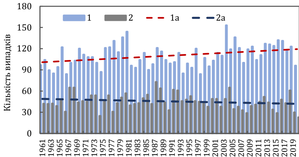
Рис. 5. Кількість днів з дощем (1) та снігом (2) зафіксованих на метеостанції Запоріжжя (1a, 2a – тренд) за період 1961–2020 рр.
