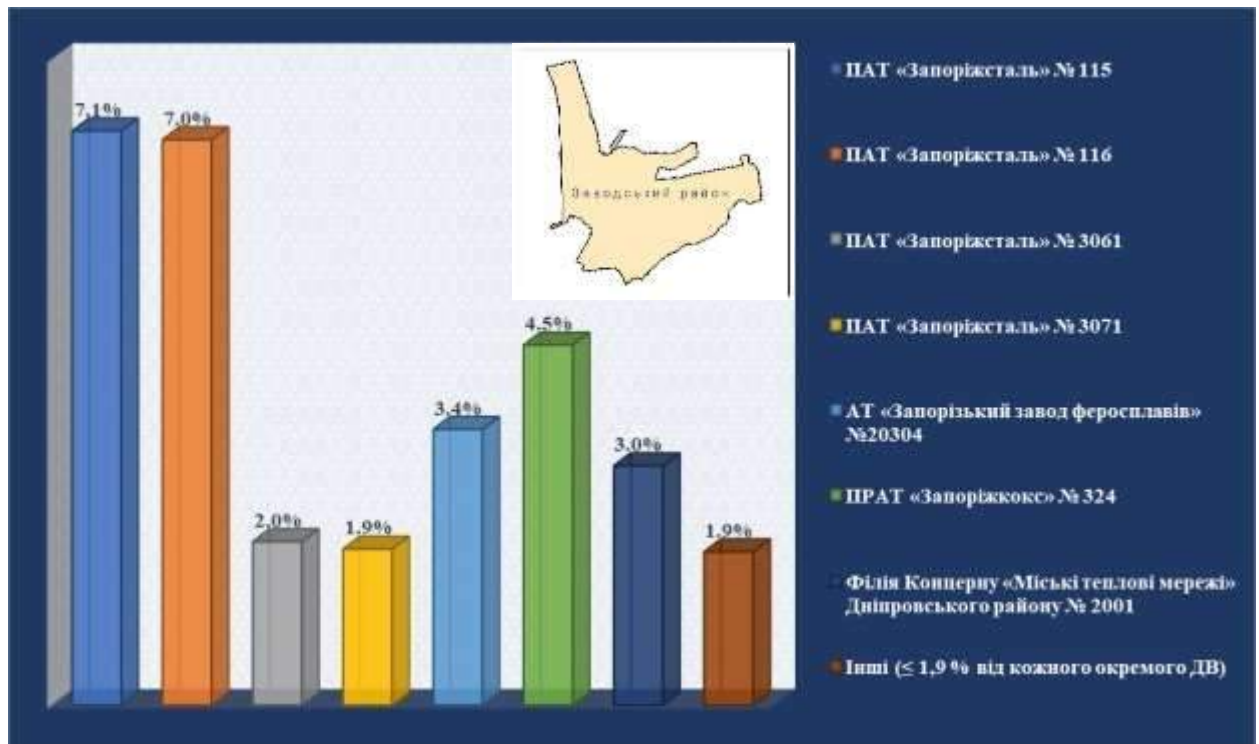
Рис. 6.7 – Внесок основних ДВ в загальне забруднення атмосферного повітря азотом діоксидом у Заводському районі
