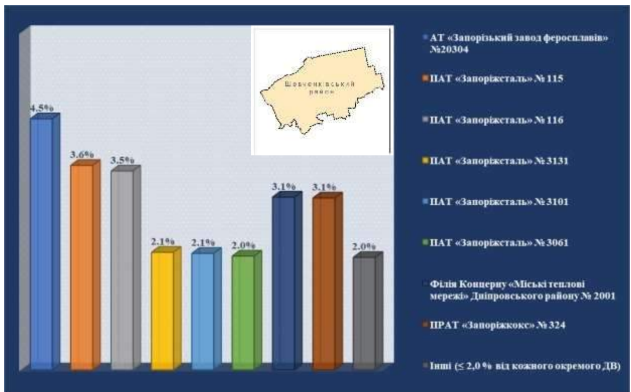
Рис. 6.10 – Внесок основних ДВ в загальне забруднення атмосферного повітря азотом діоксидом у Шевченківському районі
