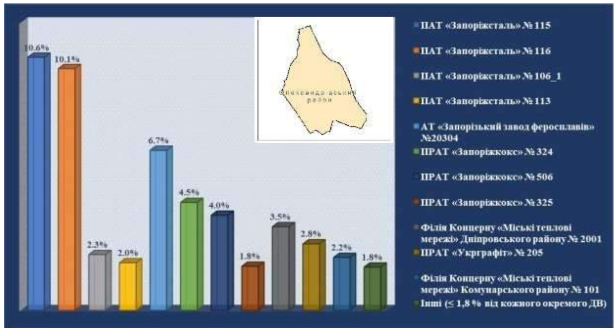
Рис. 6.11 – Внесок основних ДВ в загальне забруднення атмосферного повітря азотом діоксидом в Олександрівському районі
