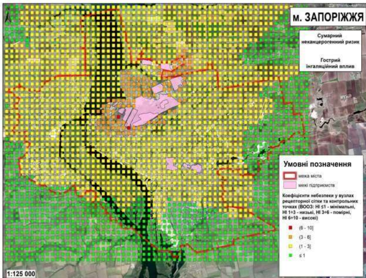
Рис. 6.1 – Рівні сумарного неканцерогенного ризику (HI) під час оцінок гострих інгаляційних впливів пріоритетних забруднюючих речовин
