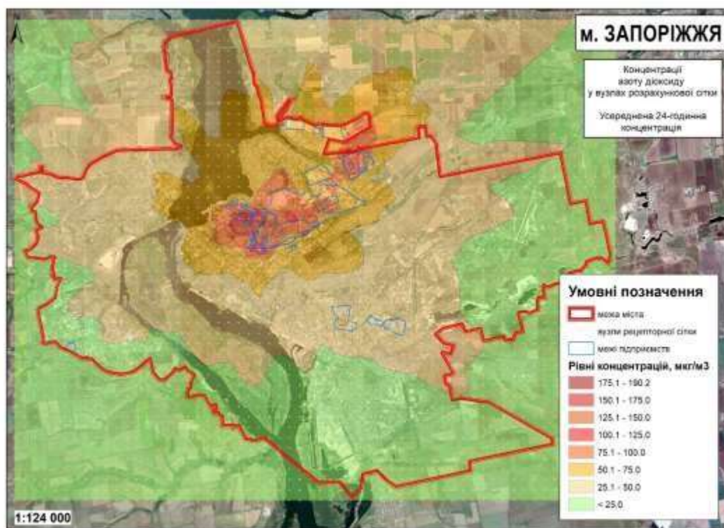
Рис. 5.15 – Результати розсіювання усереднених 24-годинних концентрацій азоту діоксиду у вузлах рецепторної сітки
