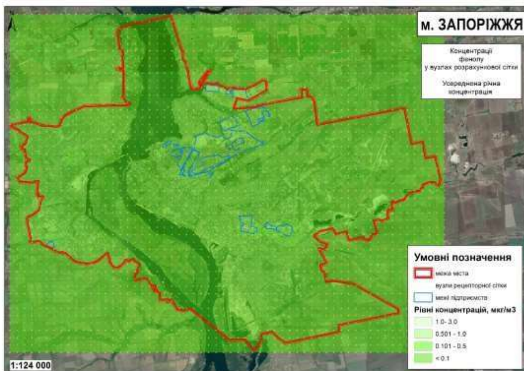
Рис. 6 – Результати розсіювання усереднених річних концентрацій фенолу у вузлах рецепторної сітки (ISC-AERMOD View, мкг/м³)
