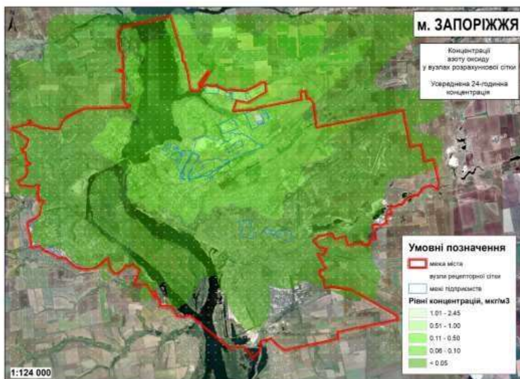
Рис. 5.16 – Результати розсіювання усереднених 24-годинних концентрацій азоту оксиду у вузлах рецепторної сітки
