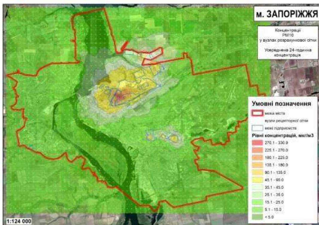
Рис. 5.12 – Результати розсіювання усереднених 24-годинних концентрацій РМ 10 у вузлах рецепторної сітки
