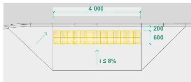
ТИП 1. Бордюрний пандус поза заокругленням перехрестя
