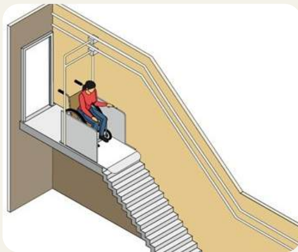
Рисунок 2.3. Схема влаштування похилого підймального пристрою на підвісах
