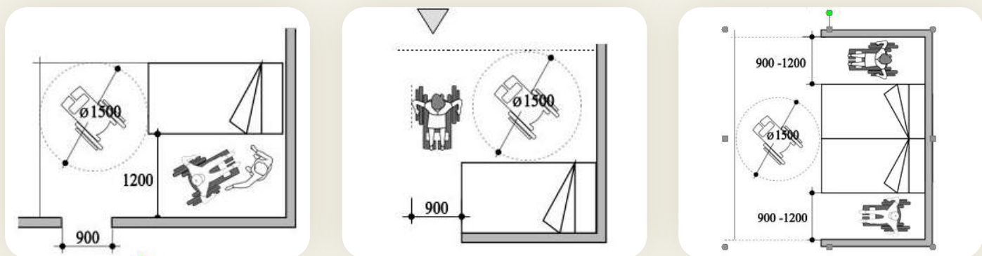
Рисунок 3.16. Схеми умеблювання спальні
