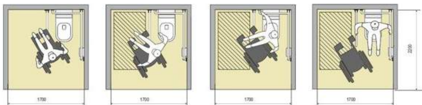
Рисунок 3.18. Способи переміщення людини між кріслом колісним та унітазом
