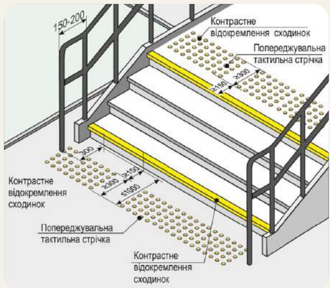
Рисунок 1.14. Облаштування сходинки
