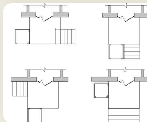
Рисунок 1.27. Взаємне розміщення підймальних пристроїв і сходів
