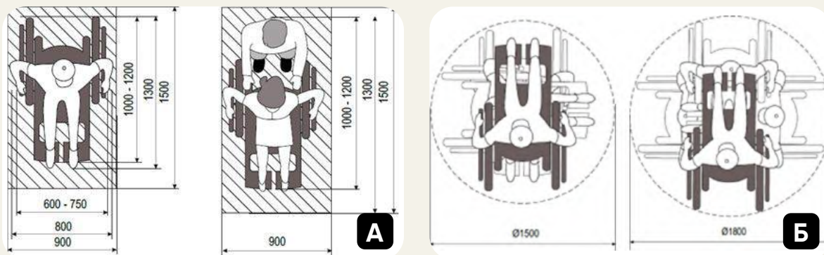
Рисунок 3.3. Простір для маневрування людей, що користуються кріслом колісним: а – мінімально допустимий; б – комфортний
