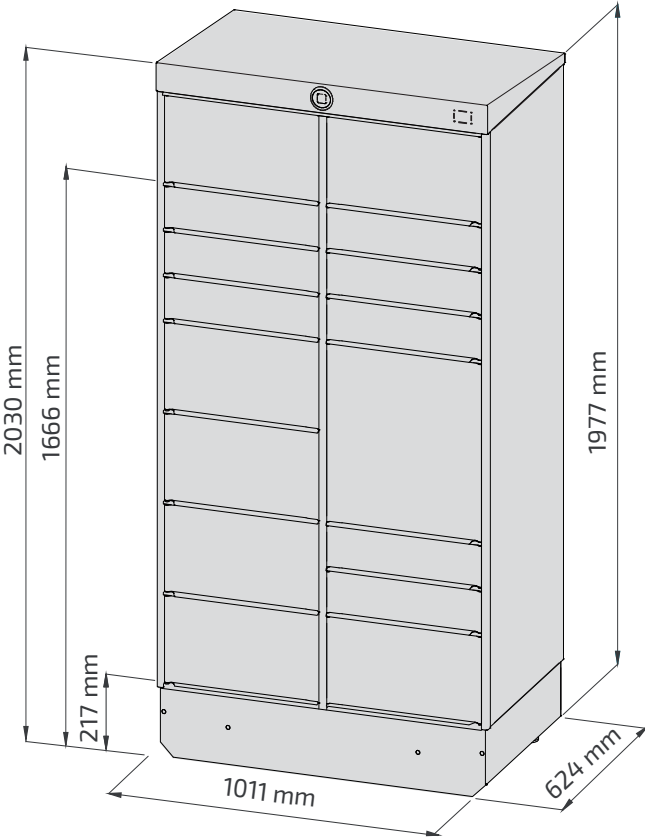
Le dimensioni esterne sono uguali per tutti i modelli
