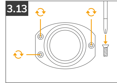
3.13 Tighten Torx screws Torx-Schrauben anziehen
