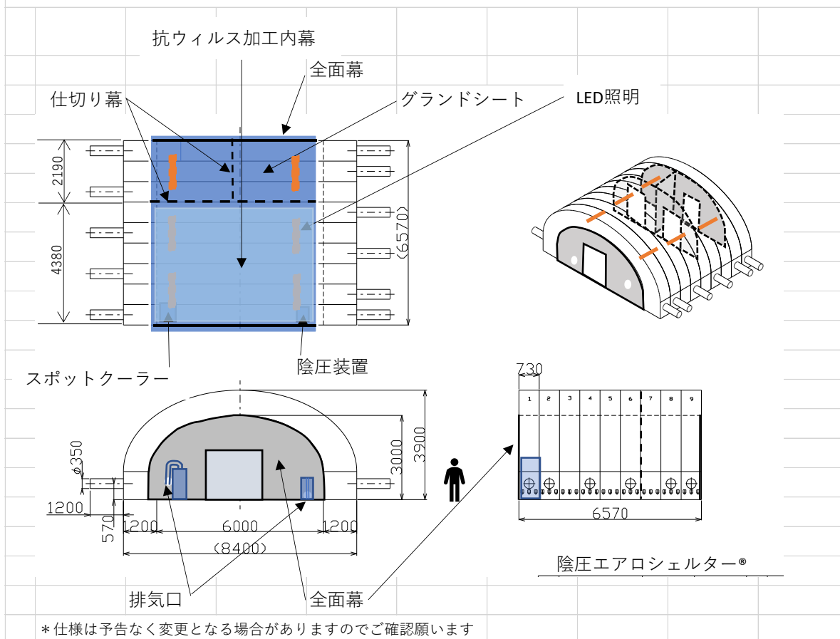
陰圧エアロシェルター®概略図
