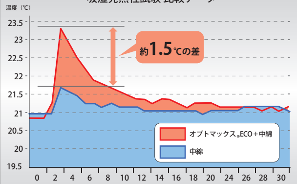
吸湿発熱性試験 比較データ
