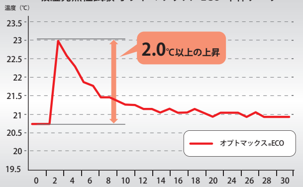
吸湿発熱性試験 オプトマックス ® ECO 単体データ
