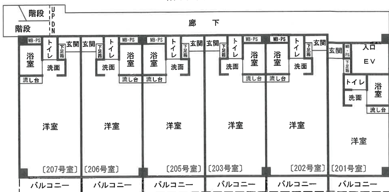
2階平面図
