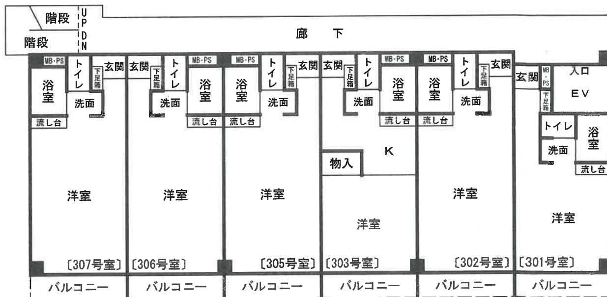
3階平面図
