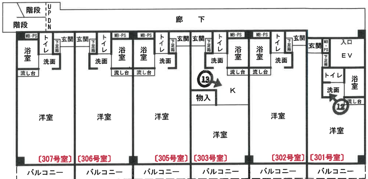
3階平面図
