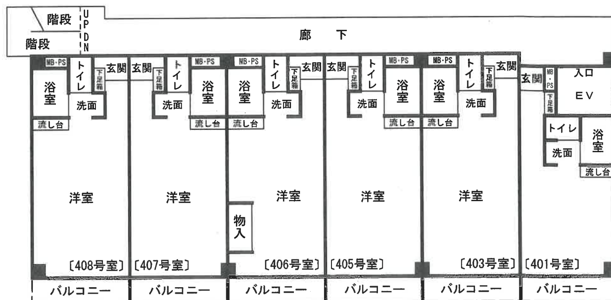
4階平面図
