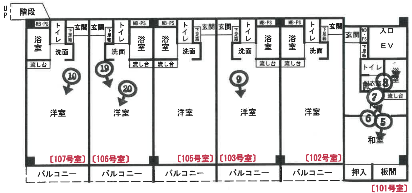
1階平面図
