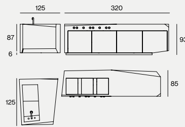
M1 320X85X93H / M2 125X125X93H
