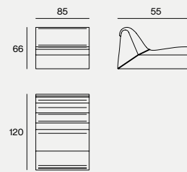
DIMENSIONS 120X85X66H
