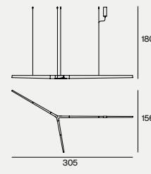
D 305X156X8H - XL B
