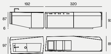
M1 320X85X93H / M2 192X97X93H
