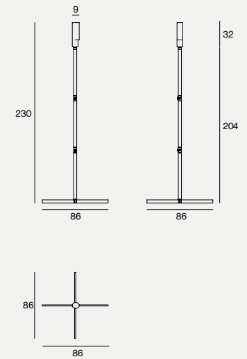
DIMENSIONS 86X86X230H
