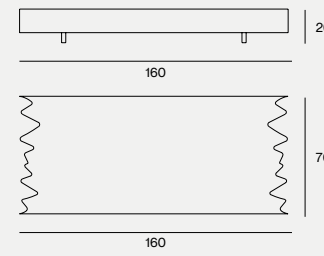
DIMENSIONS 160X70X20H
