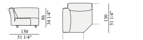
GSFA130 angolo corner angle Eckelement
