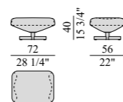
CHR015 poggiapiedi footrest ottoman Hocker
