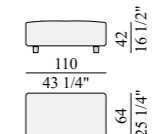
GSFPPF10 pouff pouff pouf Pouff
