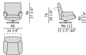
CHR010 poltrona armchair fauteuil Sessel
