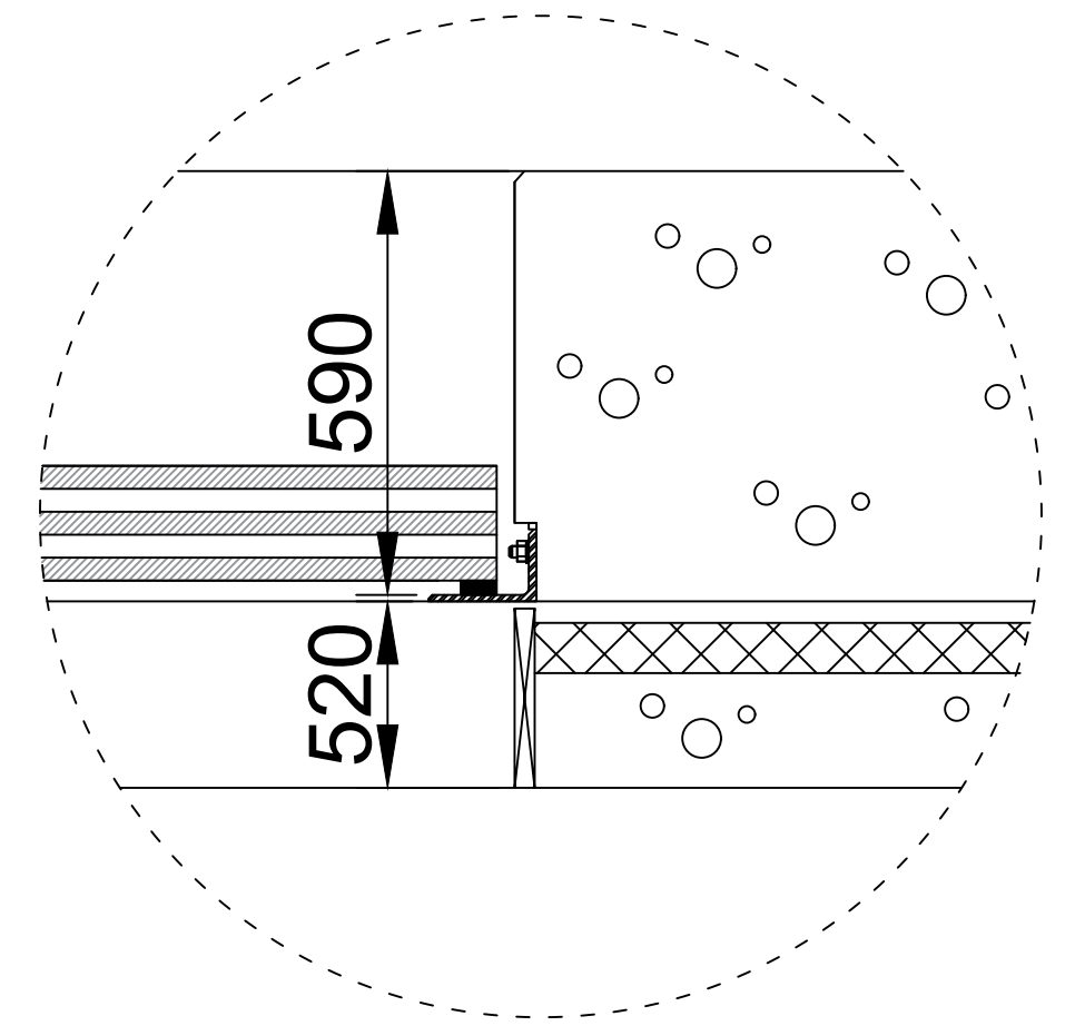
DET. 1
