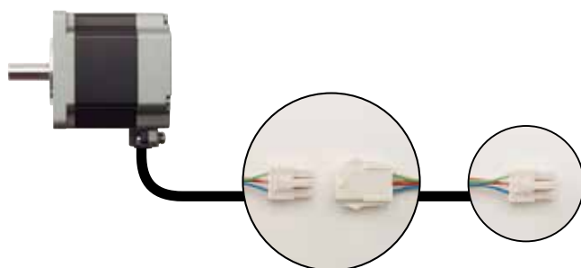
容易穿過可繞式導管和電纜線固定頭的小型馬達連接器。
