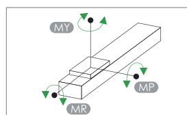
靜態容許負載慣量 Stdic Loading Moment
