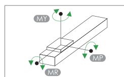
靜態容許負載慣量 Static Loading Moment
