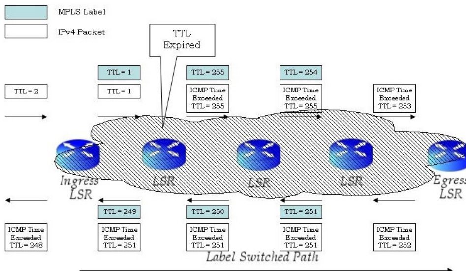
Εικόνα 2.6. Λήξη TTL εντός MPLS δικτύου
