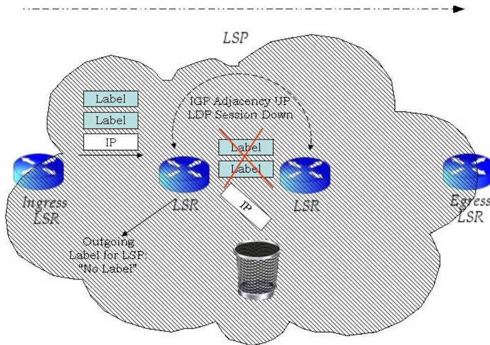
Εικόνα 3.7. Απόρριψη πακέτου λόγω μη συγχρονισμού LDP και IGP
