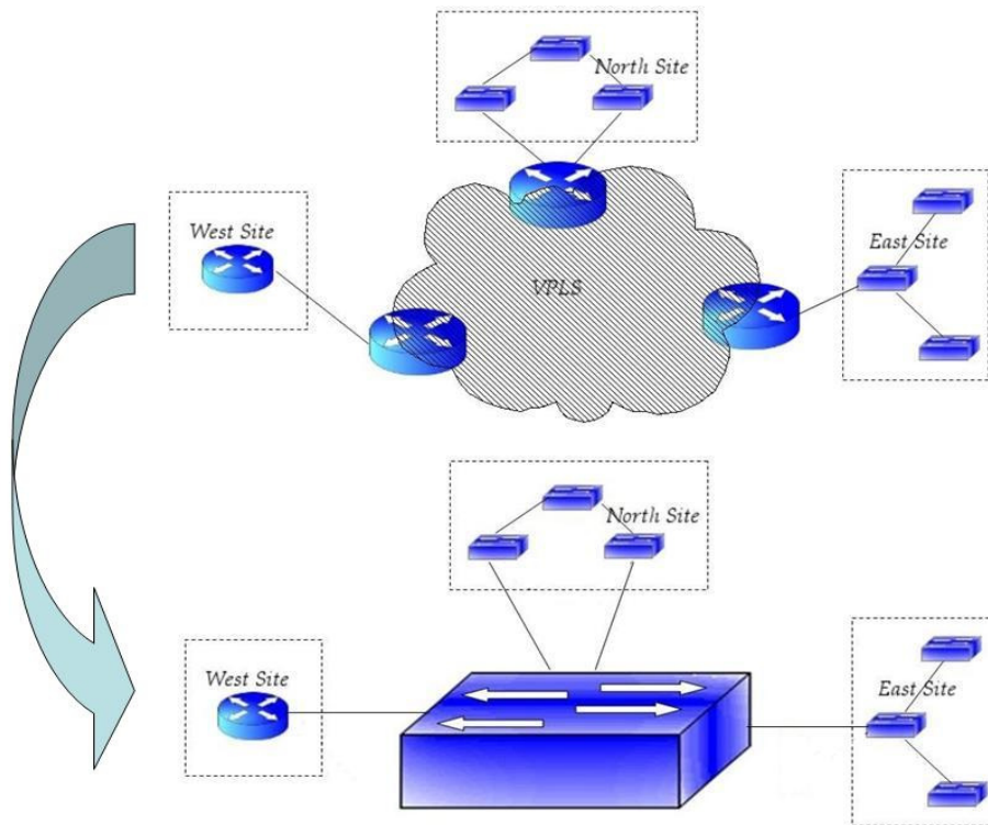
Εικόνα 1.8. Λειτουργικότητα VPLS δικτύου
