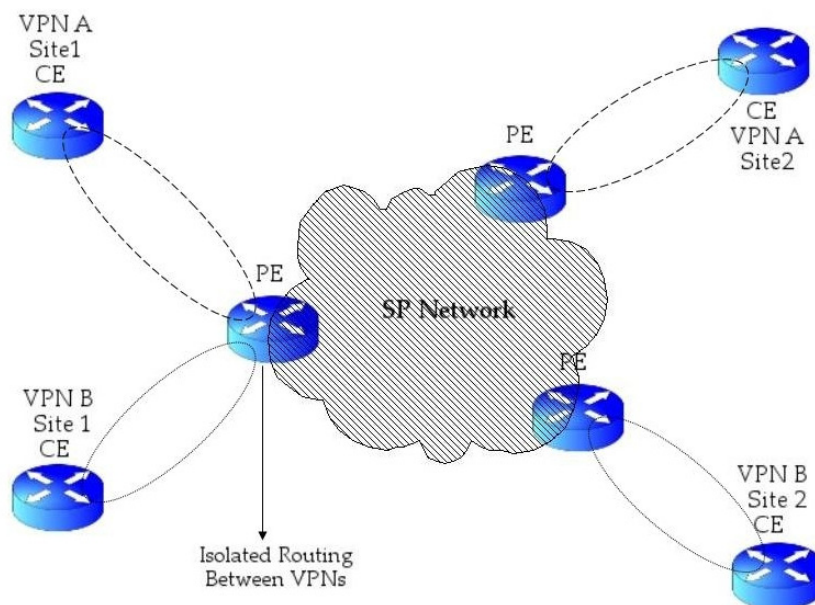
Εικόνα 5.2. Το Μοντέλο Peer VPN
