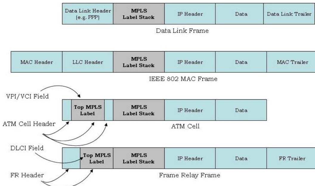
Εικόνα 1.3. Η κωδικοποίηση των ετικετών ανάλογα με την τεχνολογία 2ου επιπέδου
