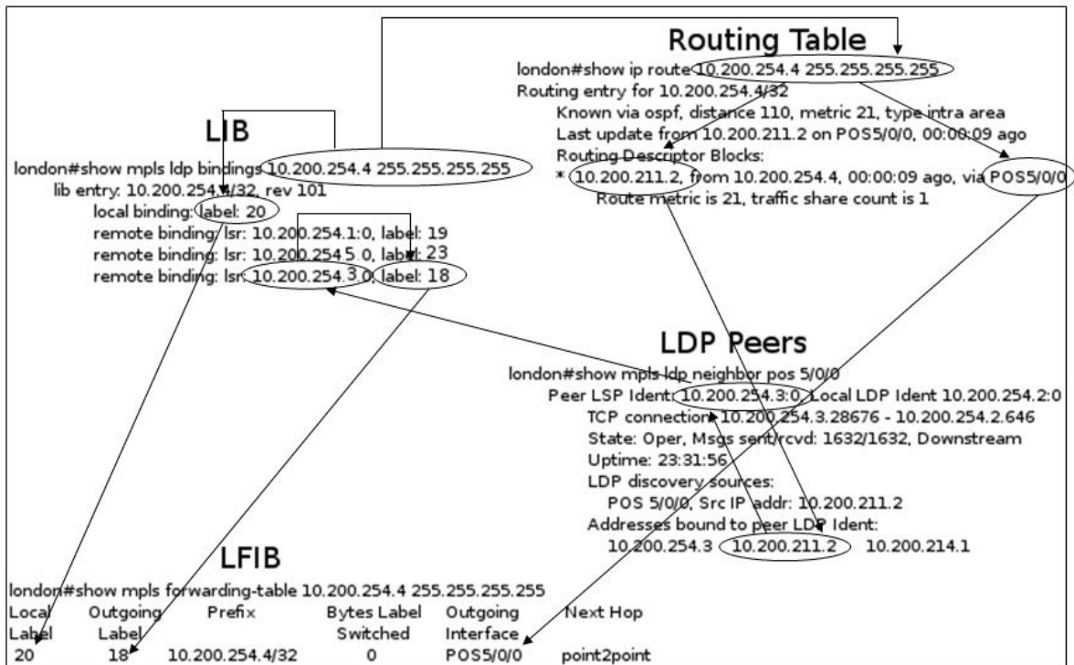
Εικόνα 3.4. Σχέση μεταξύ των πινάκων προς δημιουργία του LFIB
