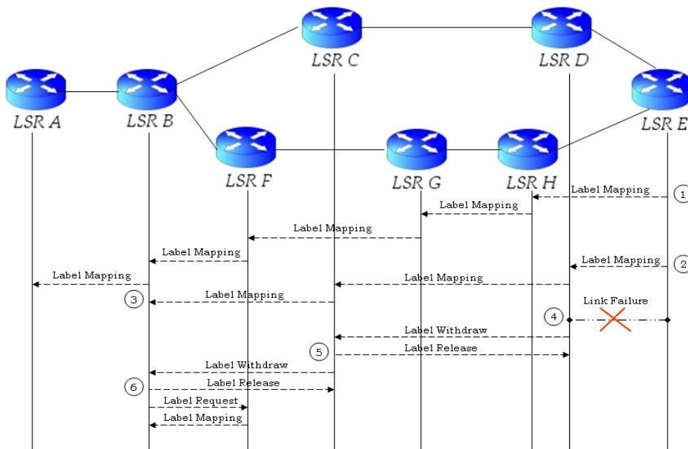
Εικόνα 3.5. Σενάριο απόσυρσης ετικετών
