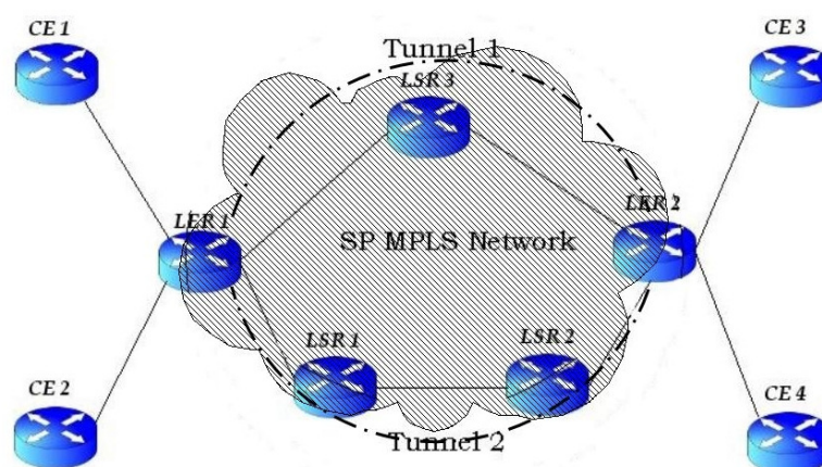
Εικόνα 4.2. MPLS δίκτυο με TE Tunnel
