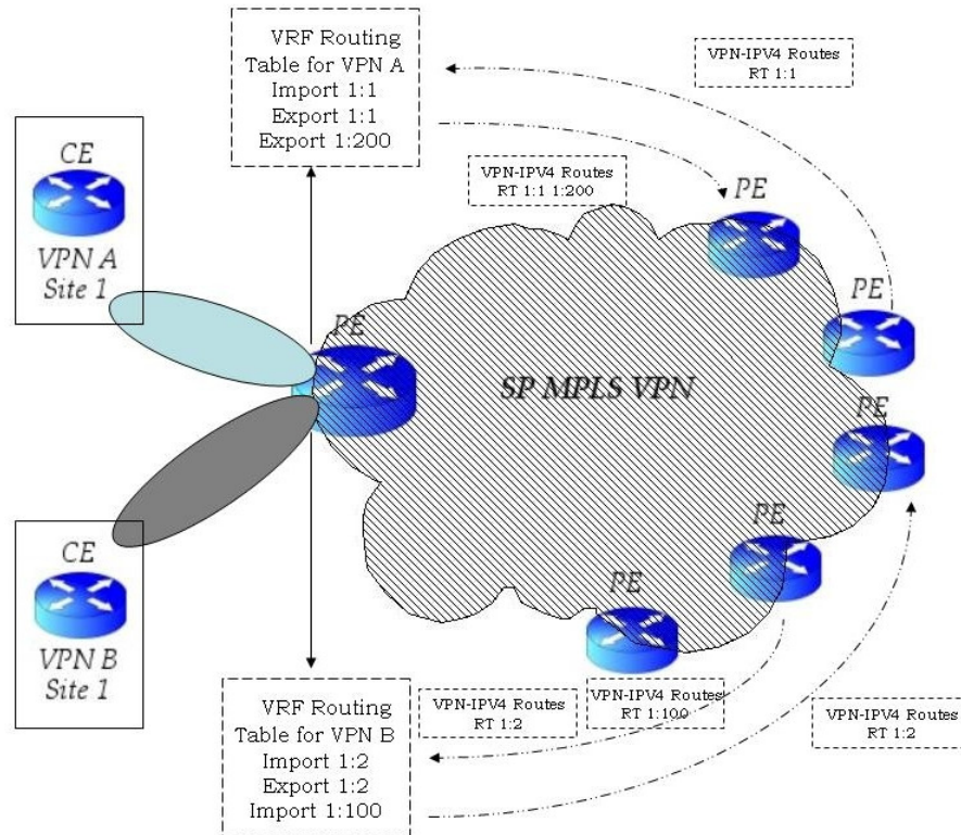
Εικόνα 5.5. Εισαγωγή και εξαγωγή RT 1
