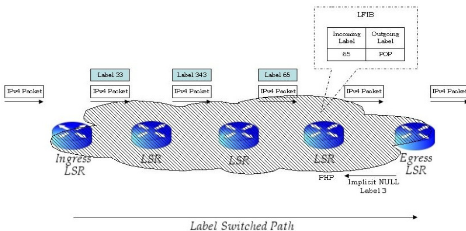
Εικόνα 2.3. Η μέθοδος PHP
