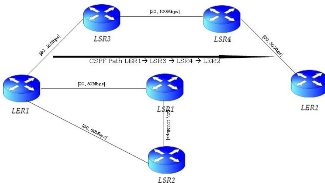
Εικόνα 4.7. Εύρεση διαδρομής σύμφωνα με τον CSPF αλγόριθμο
