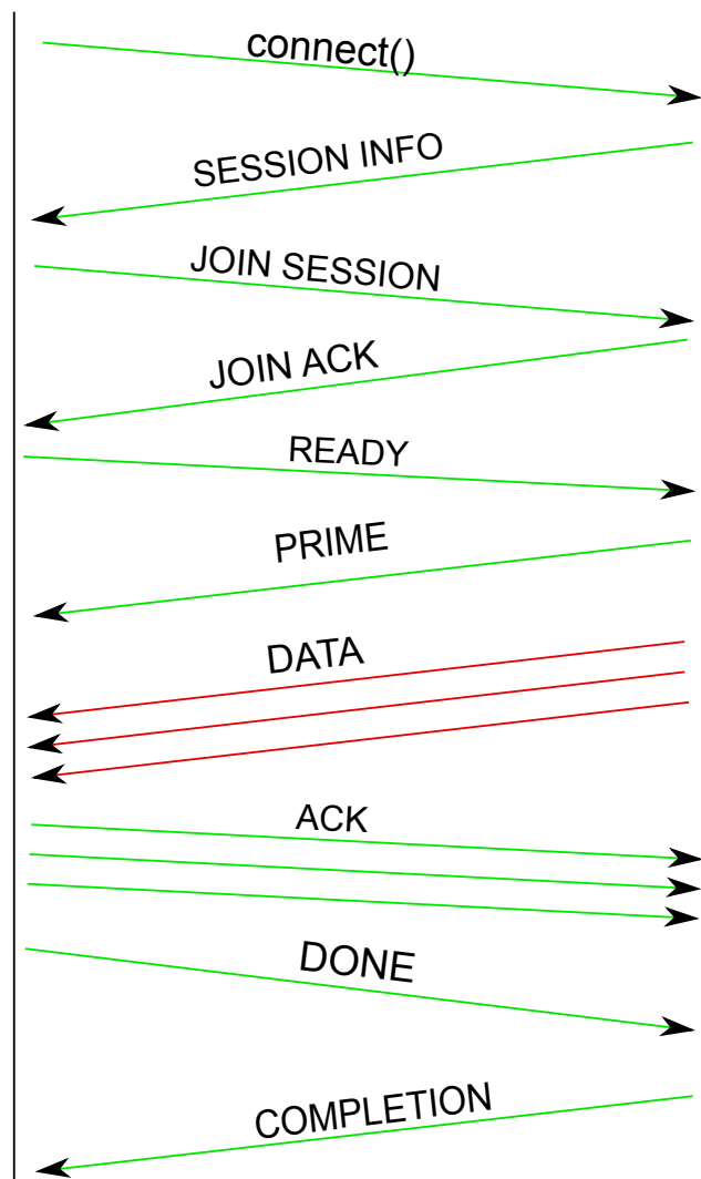
Figure 2.4: Ανταλλαγή μηνυμάτων μεταξύ sender - receiver
