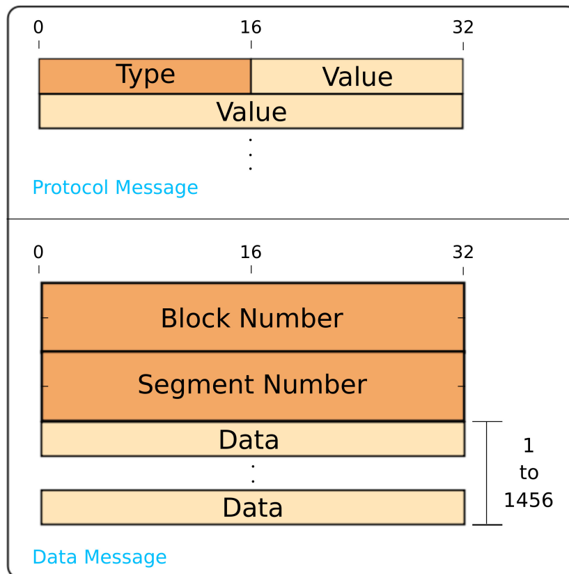
Figure 4.1: Μορφή Μηνυμάτων
