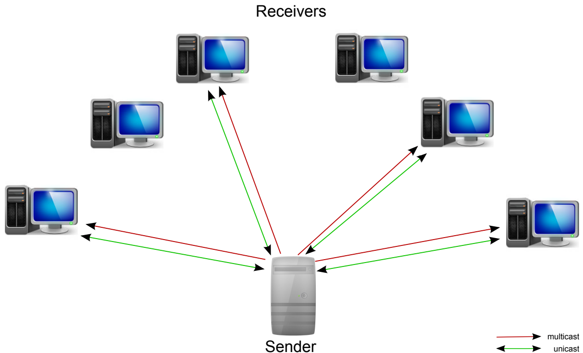
Figure 2.1: Μοντέλο αποστολής
