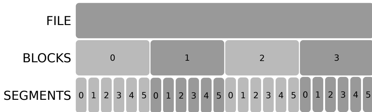
Figure 2.5: Χωρισμός αρχείου
