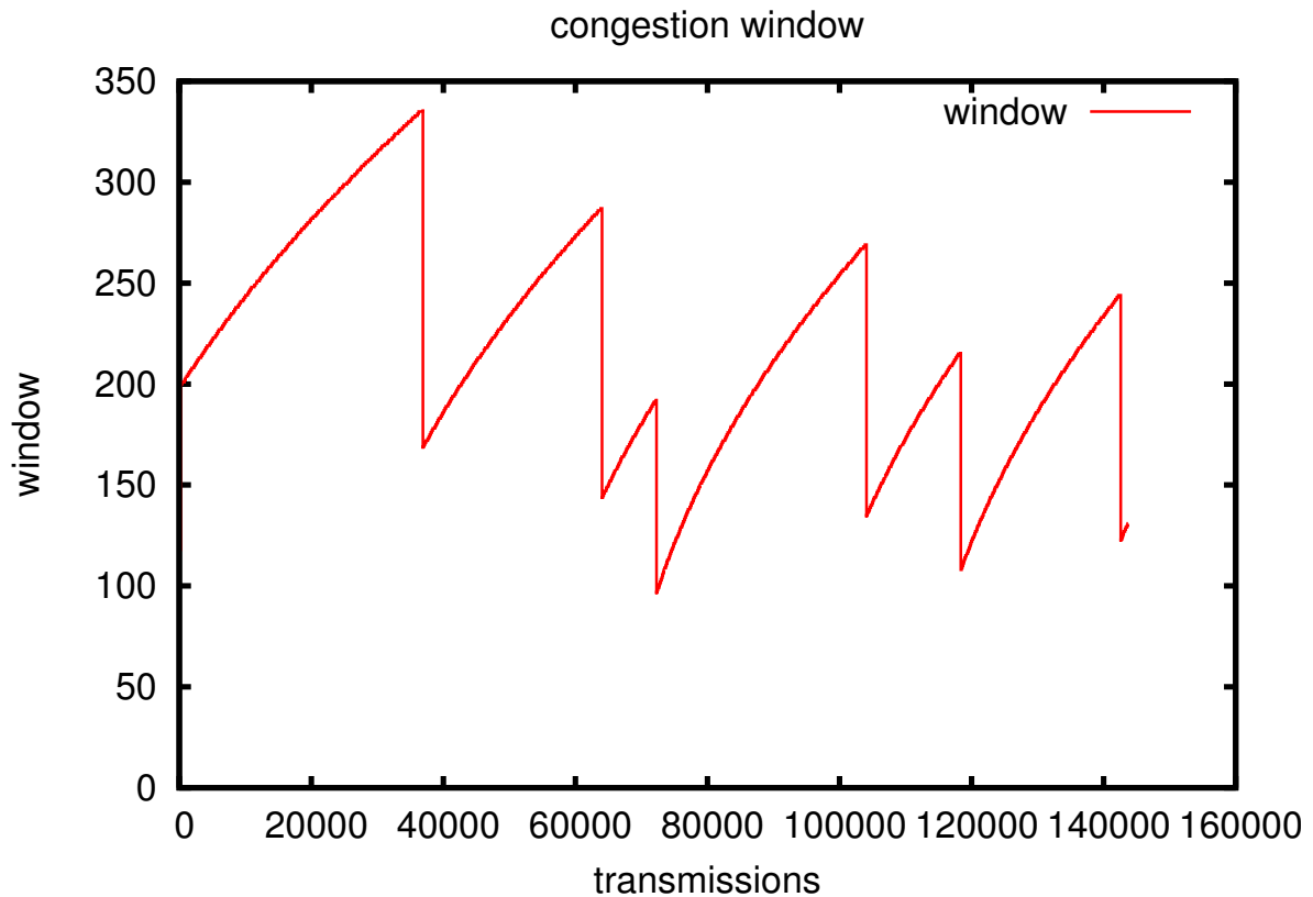
Figure 3.3: Παράθυρο συμφόρησης
