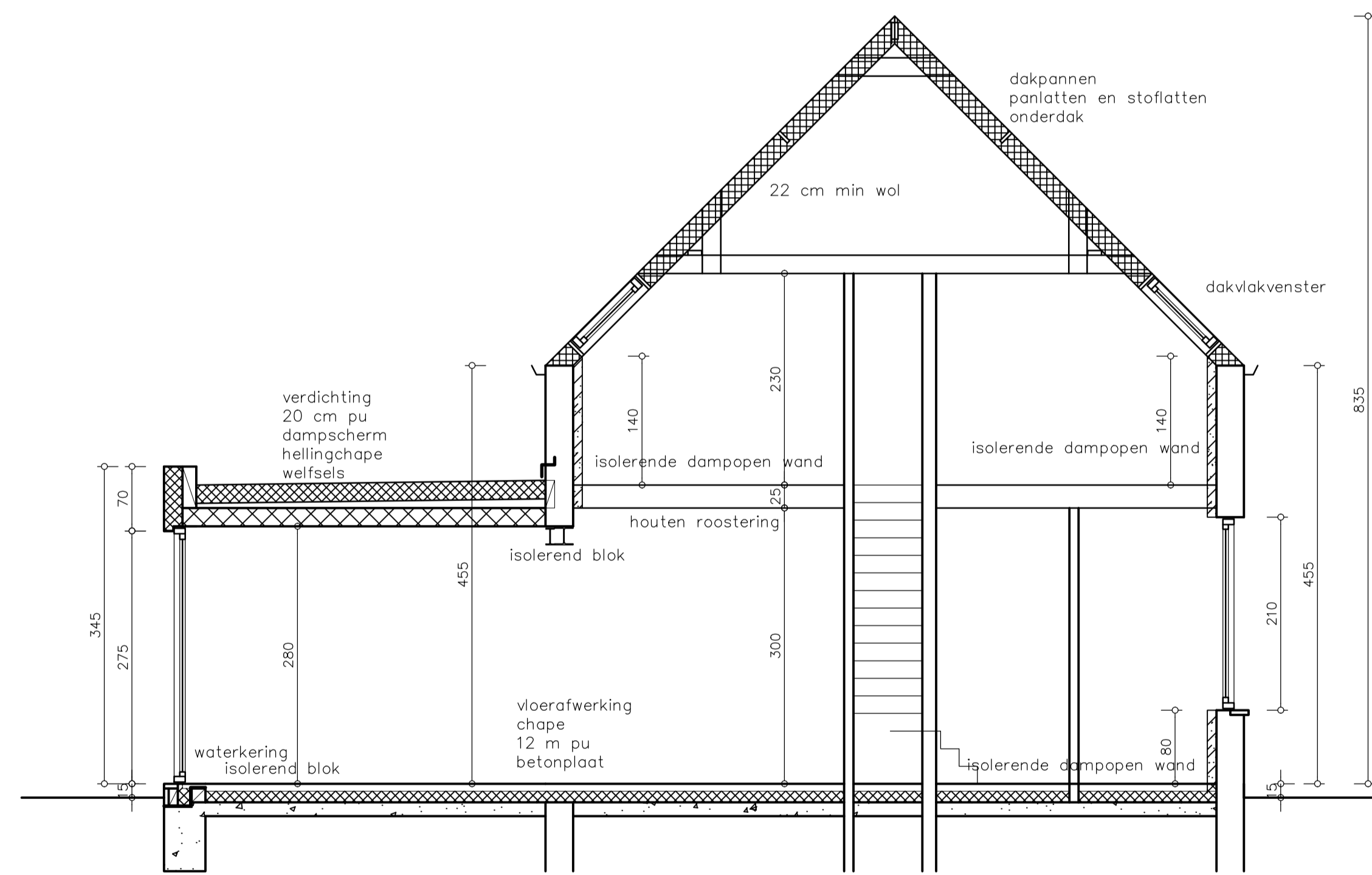
doorsnede A woning arbeiderswoningen
