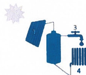
1. Zonnecollector | 2. Opslagvat zonneboiler | 3. Sanitair warm water | 4. Afgifteenheid voor ruimteverwarming (optioneel)
