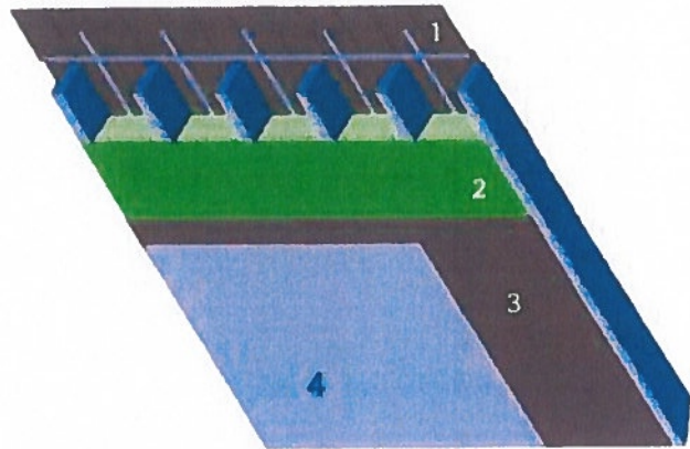
1. Onderdak | 2. Isolatie | 3. Dampschermelement | 4. binnenafwerking
