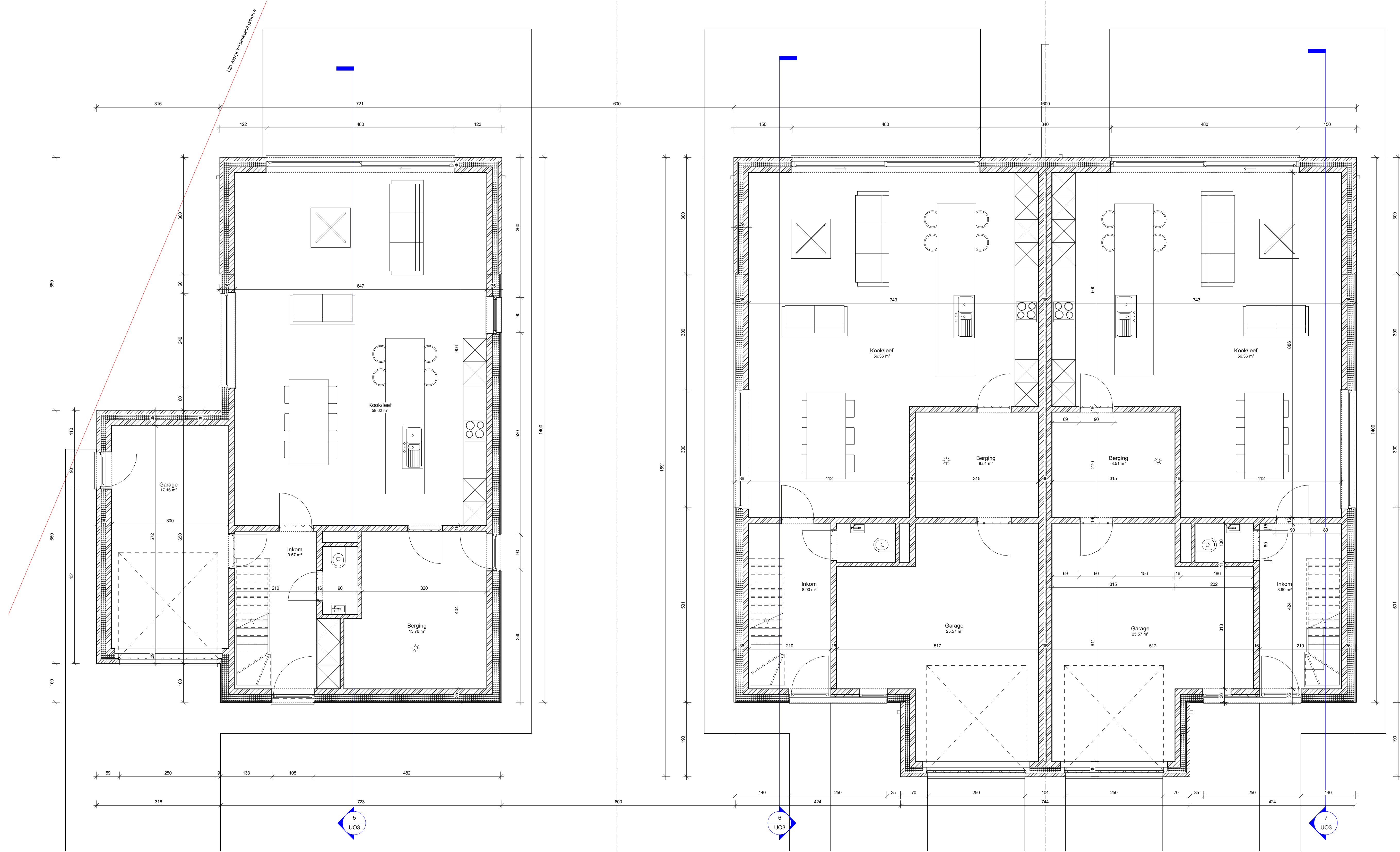
1 00 Plan gelijkvloers 1/50
