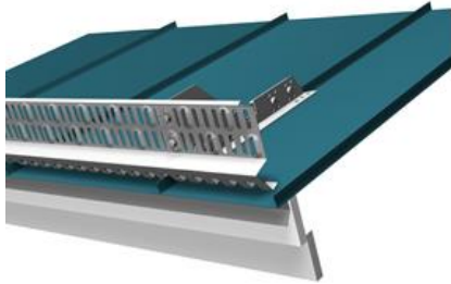
Kuva 1. VARMA 180 konesaumakatolle
