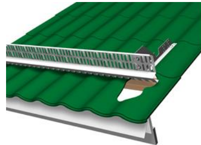
Kuva 2. VARMA 180 tiilikatolle
