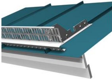
Kuva 1. VARMA 180 konesaumakatolle
