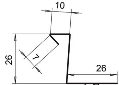
Kuva 2. Klammerin mittakuva
