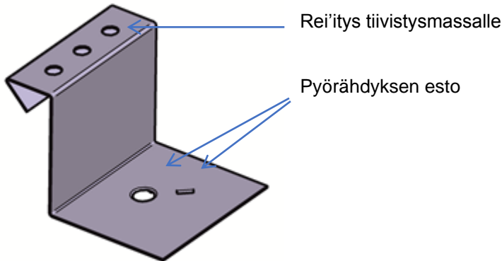
Kuva 1. Klammeri rei'illä
