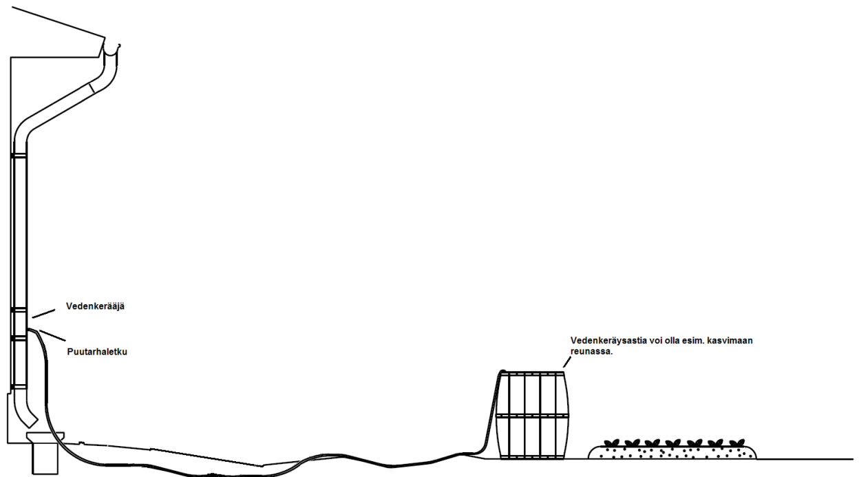
Kuva 2. Vedenkerääjän toimintaperiaate
