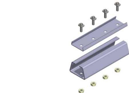
Kuva 9. Vaakakiskon ulkopuolinen jatkos
