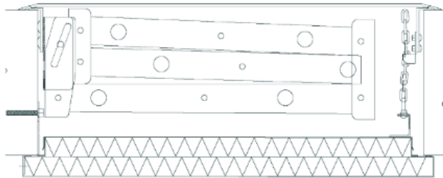
Kuva 5. Palokatkollisen parvekeluukun läpileikkaus
