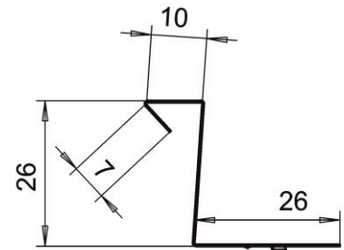
Kuva 2. Klammerin mittakuva
